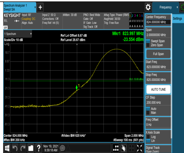
Band5-10MHz-QPSK-20450-1RB#0
