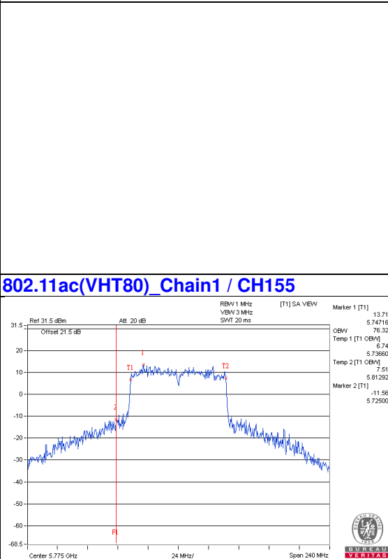
802.11ac(VHT80)_Chain1 / CH155
