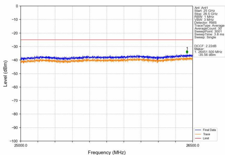
Band41_20MHz_QPSK_LCH_2506MHz_RB_100_0_NTNV
