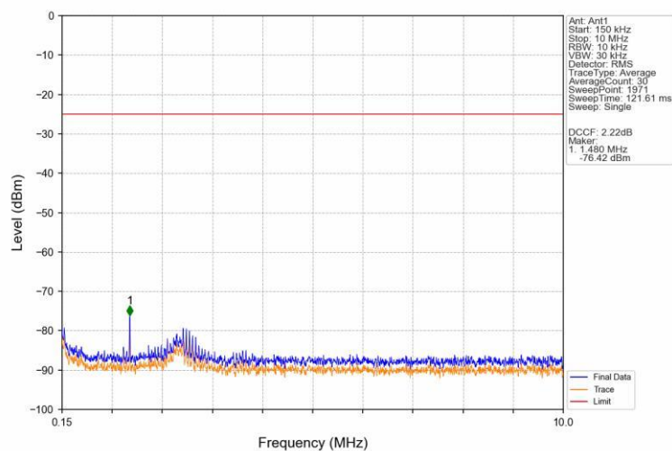
Band41 20MHz 16QAM MCH 2593MHz RB 1 0 NTNV
