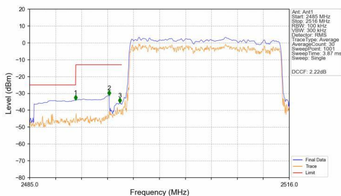
Band41_20MHz_QPSK_LCH_2506MHz_RB_100_0_NTNV
