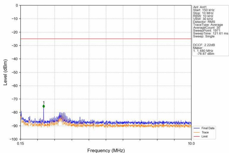
Band41_20MHz_QPSK_LCH_2506MHz_RB_1_0_NTNV
