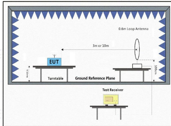
9KHz~30MHz
