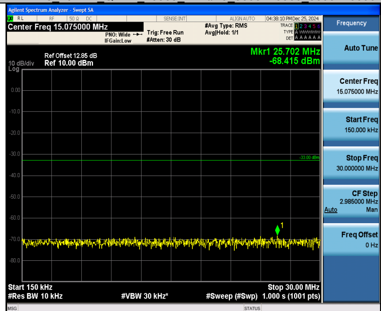
Band25 10MHz 16QAM 26365 1RB#49 0.15~30 0.15~30
