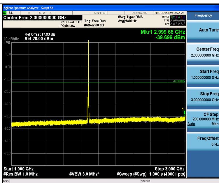
Band25 10MHz QPSK 26365 1RB#49 1000~3000 1000~3000
