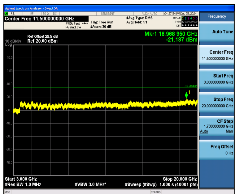
Band25 10MHz QPSK 26365 1RB#49 3000~20000 3000~20000
