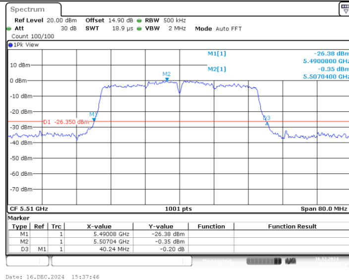
11N40MIMO_Ant2_5510
