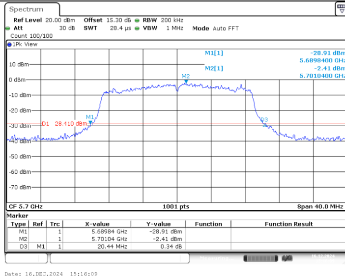
11N20MIMO_Ant2_5700
