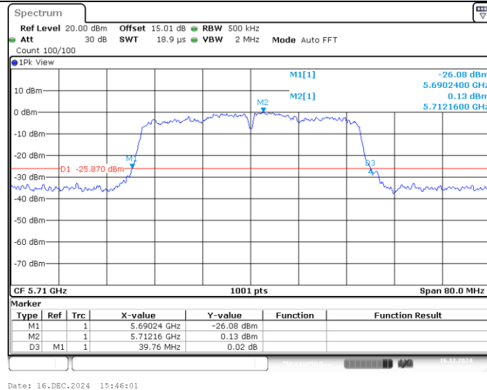
11N40MIMO_Ant2_5710
