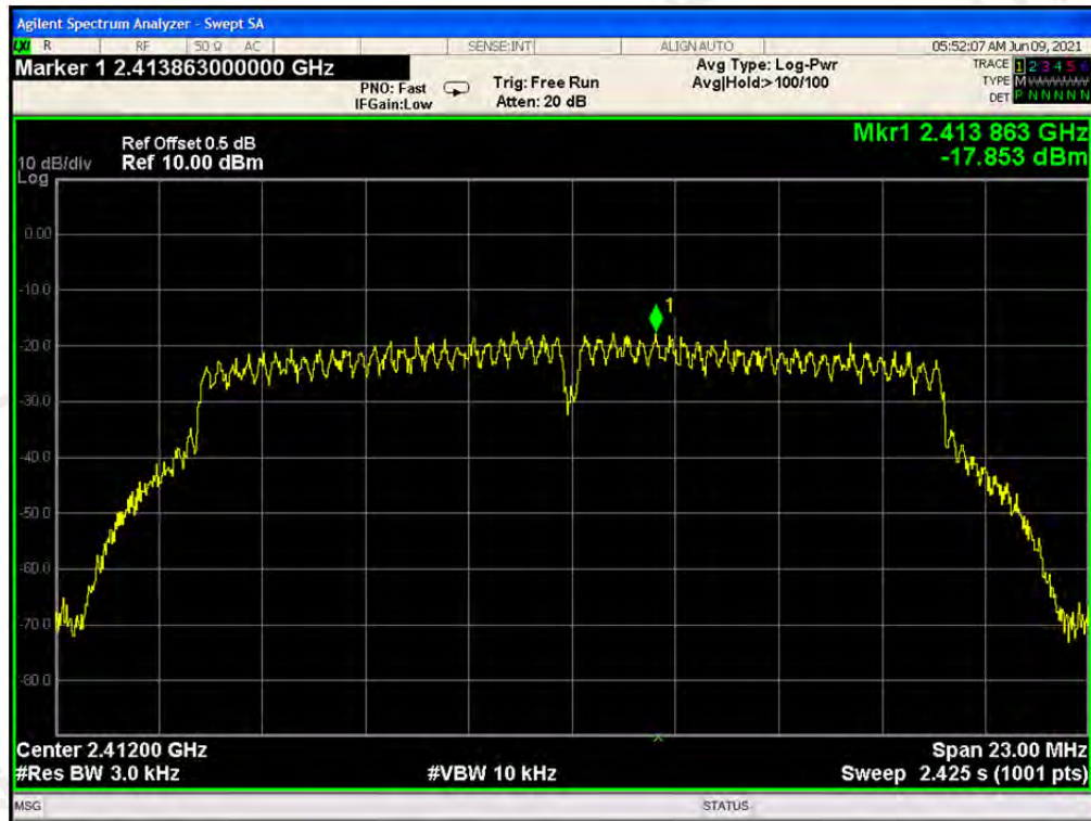
CH1: 2412MHz-ANT1
