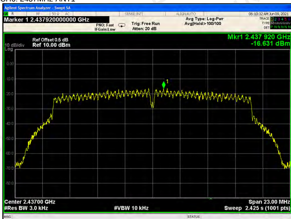
CH6: 2437MHz-ANT1
