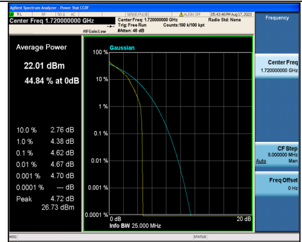
Band4-20MHz-QPSK-20050-1RB#0-PASS
