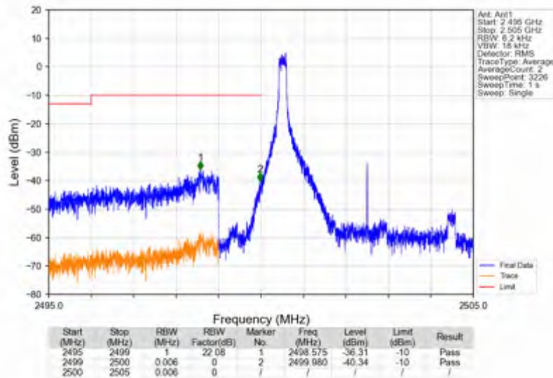
n7_15kHz_SISO_NTV_5MHz_CP-OFDM QPSK_2502.5MHz_Inner_1RB_Left
