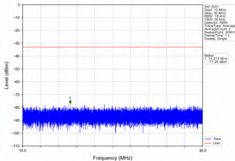
n7_15kHz_SISO_NTNV_20MHz_CP-OFDM QPSK_2510MHz_Inner_1RB_Left
