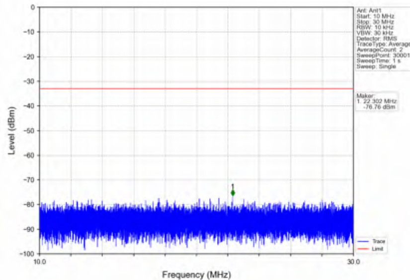
n7_15kHz_SISO_NTNV_20MHz_DFT-s-OFDM PI/2 BPSK_2510MHz_Edge_1RB_Left
