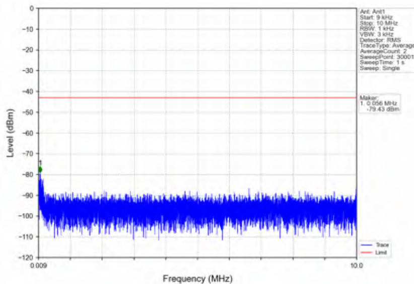
n7_15kHz_SISO_NTNV_10MHz_DFT-s-OFDM_PI/2_BPSK_2505MHz_Inner_1RB_Left
