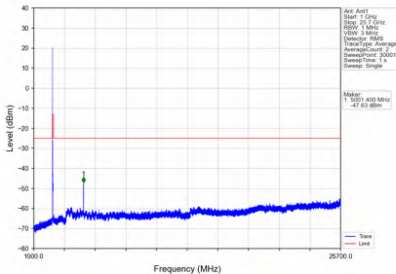
n7_15kHz_SISO_NTNV_20MHz_CP-OFDM QPSK_2535MHz_Edge_1RB_Left
