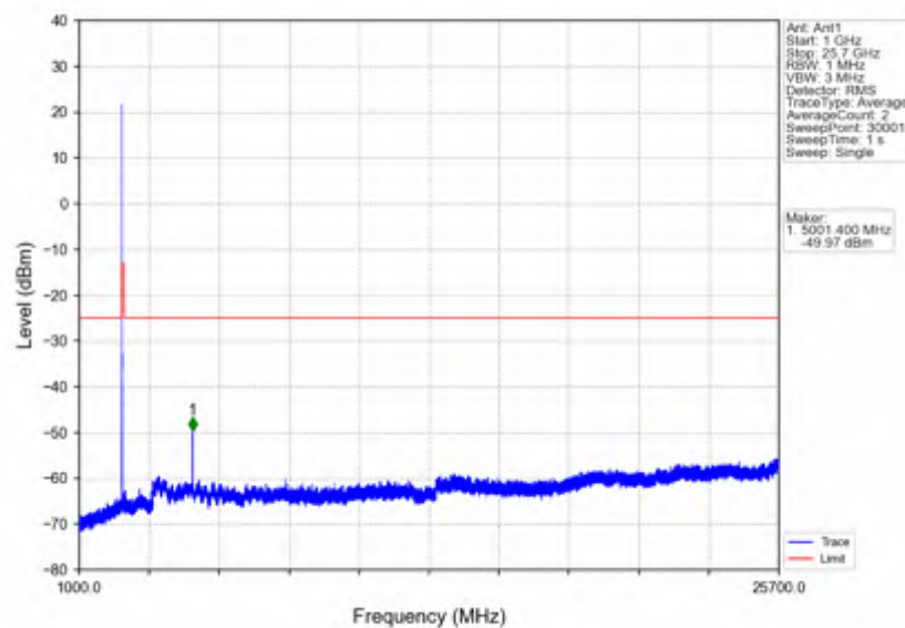
n7_15kHz_SISO_NTNV_10MHz_DFT-s-OFDM QPSK_2505MHz_Inner_1RB_Left
