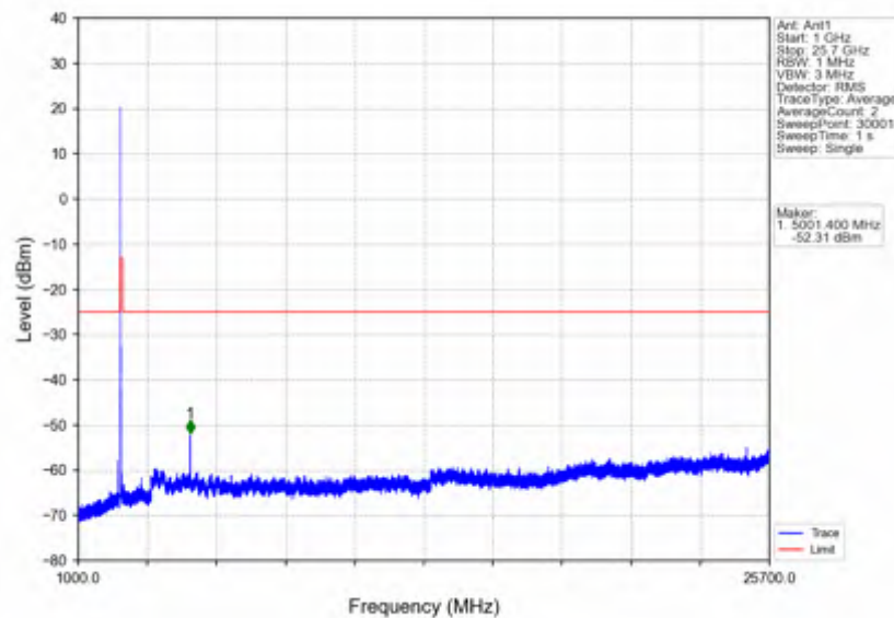
n7 15kHz SISO NTN 15MHz DFT-s-OFDM QPSK 2507.5MHz Edge 1RB Left
