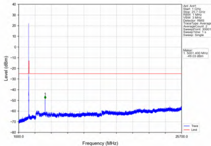
n7_15kHz_SISO_NTNV_20MHz_DFT-s-OFDM_QPSK_2510MHz_Inner_1RB_Left
