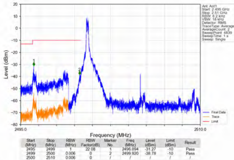
n7_15kHz_SISO_NTNV_10MHz_DFT-s-OFDM_PI/2_BPSK_2505MHz_Inner_1RB_Left
