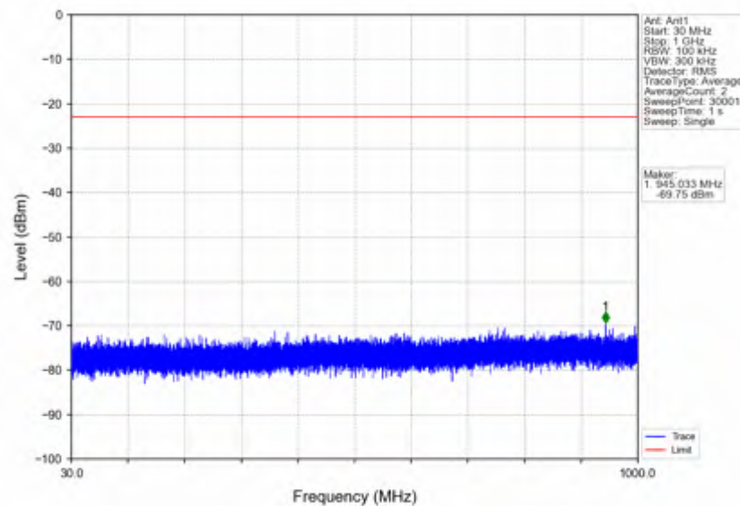
n7 15kHz SISO NTNV 10MHz CP-OFDM QPSK 2535MHz Edge 1RB Left
