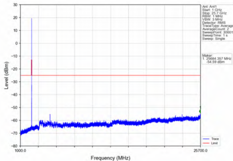
n7 15kHz SISO NTNV 10MHz CP-OFDM QPSK 2535MHz Edge 1RB Left
