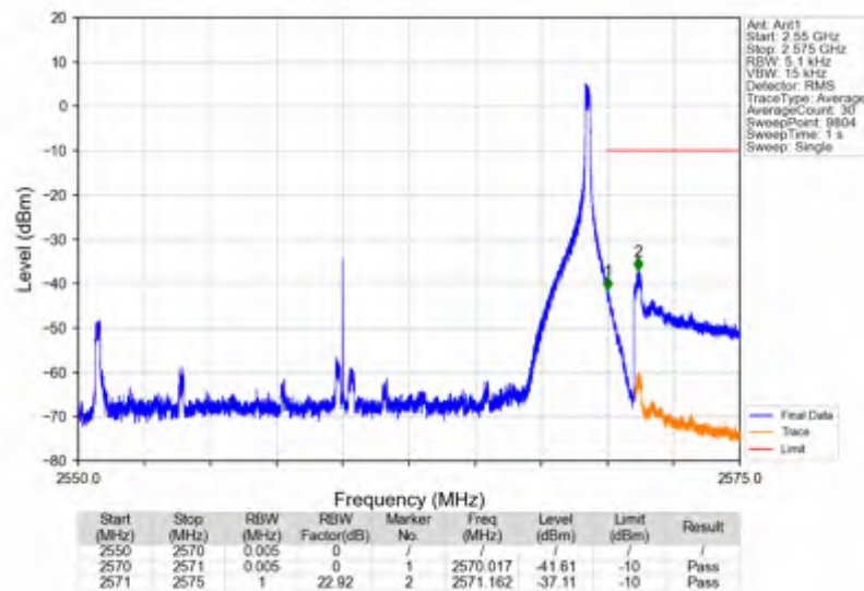
n7_15kHz_SISO_NTNV_20MHz_DFT-s-OFDM QPSK_2560MHz_Inner_1RB_Right
