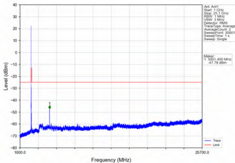
n7_15kHz_SISO_NTNV_20MHz_DFT-s-OFDM PI/2 BPSK_2535MHz_Edge_1RB_Left
