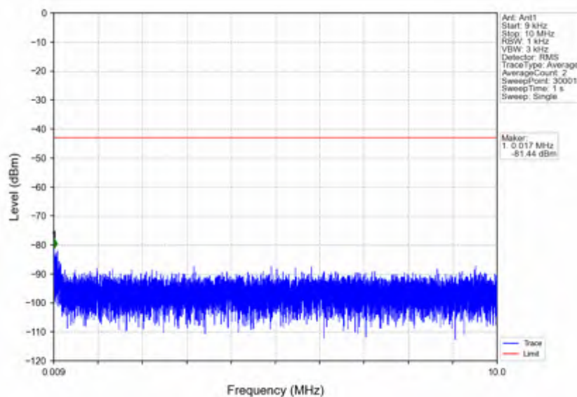
n7_15kHz_SISO_NTNV_20MHz_DFT-s-OFDM_PI/2_BPSK_2510MHz_Edge_1RB_Left
