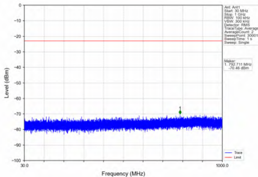
n7_15kHz_SISO_NTNV_10MHz_DFT-s-OFDM QPSK_2505MHz_Inner_1RB_Left
