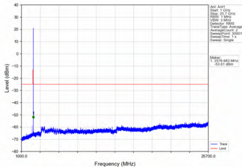
n7 15kHz SISO NTN 5MHz DFT-s-OFDM QPSK 2567.5MHz Edge 1RB Right
