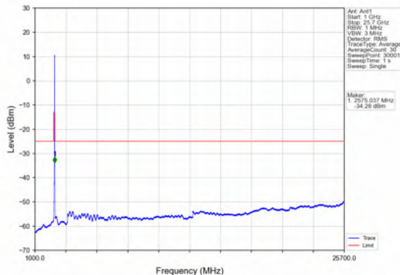
n7_15kHz_SISO_NTNV_20MHz_DFT-s-OFDM QPSK_2560MHz_Inner_1RB_Right
