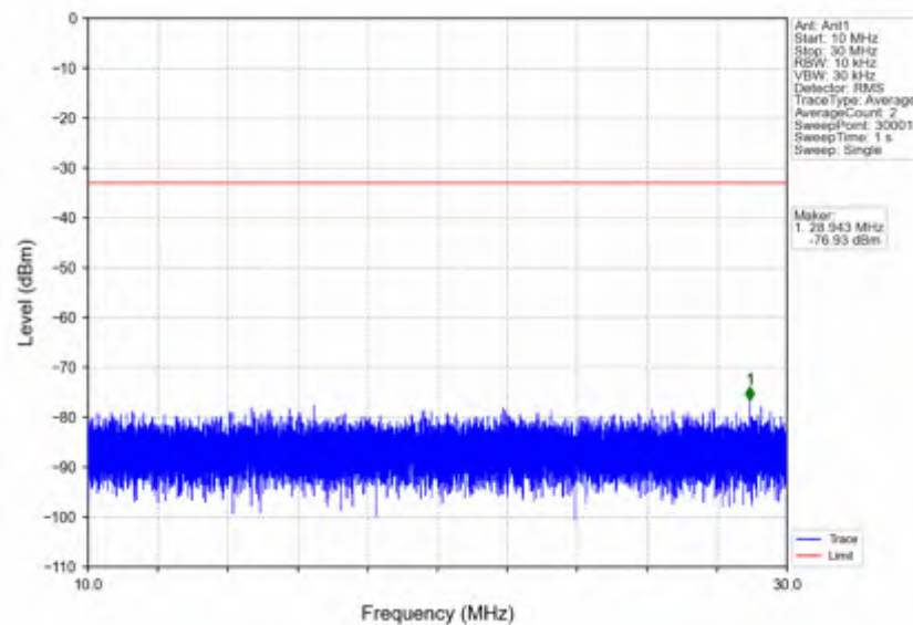
n7_15kHz_SISO_NTNV_20MHz_CP-OFDM QPSK_2535MHz_Edge_1RB_Left
