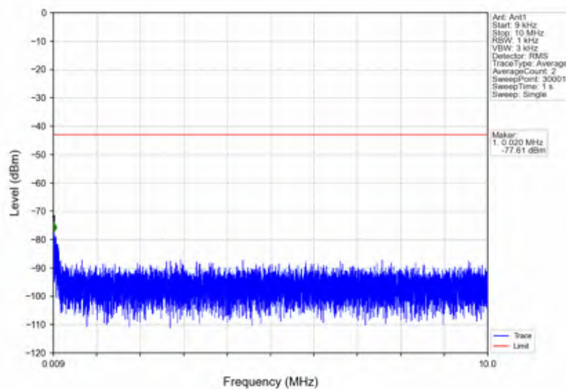
n7_15kHz_SISO_NTNV_20MHz_CP-OFDM_QPSK_2510MHz_Inner_1RB_Left
