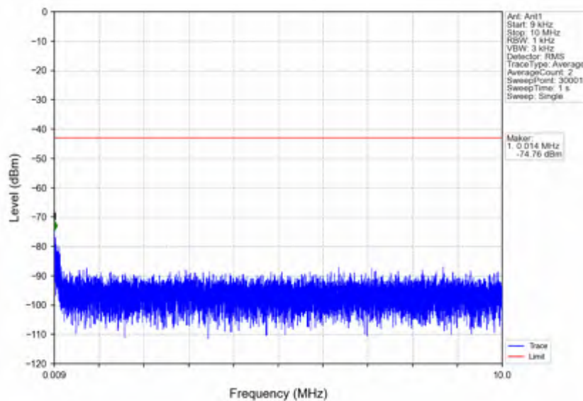
n7_15kHz_SISO_NTNV_10MHz_CP-OFDM_QPSK_2505MHz_Inner_1RB_Left
