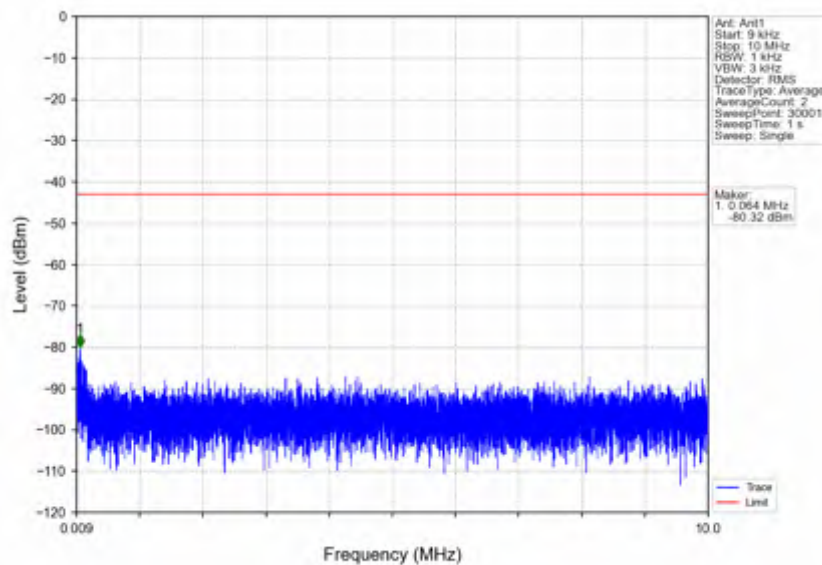
n7_15kHz_SISO_NTNV_20MHz_DFT-s-OFDM PI/2 BPSK_2510MHz_Inner_1RB_Left
