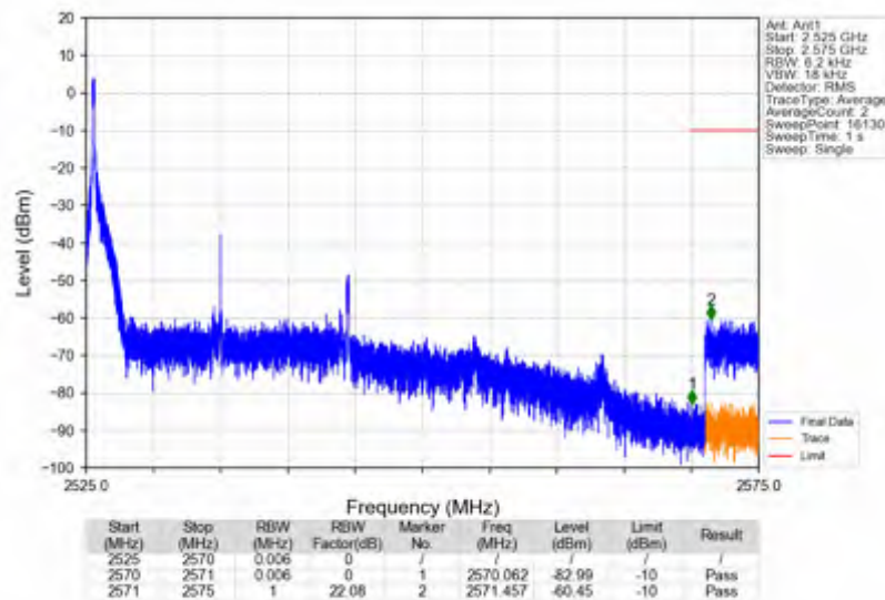
n7_15kHz_SISO_NTNV_20MHz_CP-OFDM QPSK_2535MHz_Edge_1RB_Left
