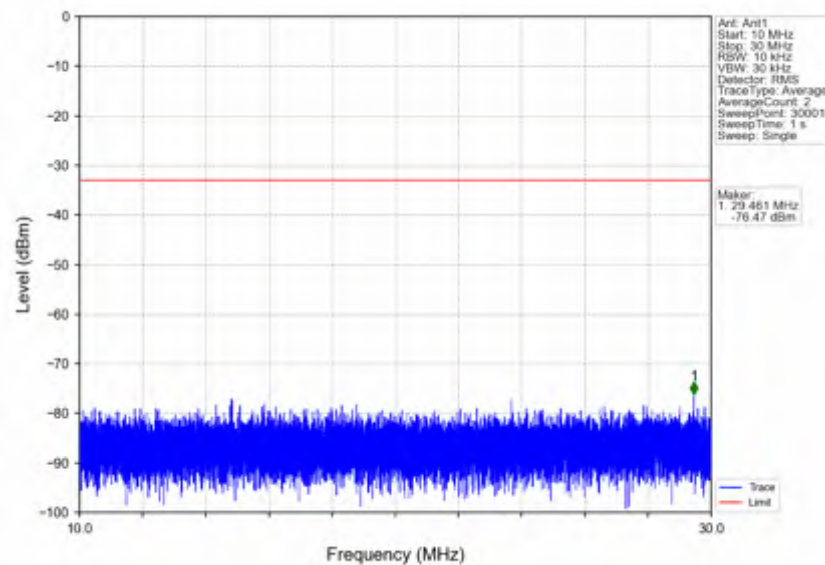
n7_15kHz_SISO_NTNV_20MHz_DFT-s-OFDM QPSK_2510MHz_Edge_1RB_Left
