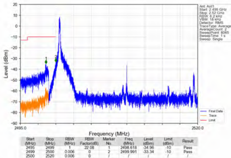
n7_15kHz_SISO_NTNV_20MHz_DFT-s-OFDM_PI/2_BPSK_2510MHz_Edge_1RB_Left
