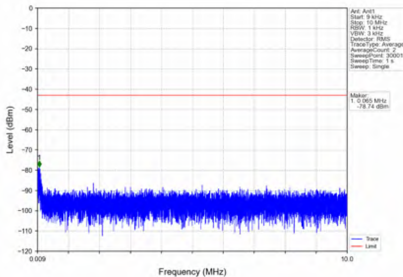
n7_15kHz_SISO_NTV_5MHz_CP-OFDM QPSK_2502.5MHz_Inner_1RB_Left
