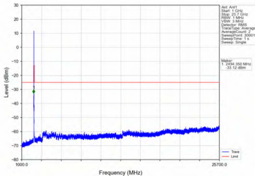
n7_15kHz_SISO_NTNV_20MHz_DFT-s-OFDM_QPSK_2510MHz_Inner_1RB_Left
