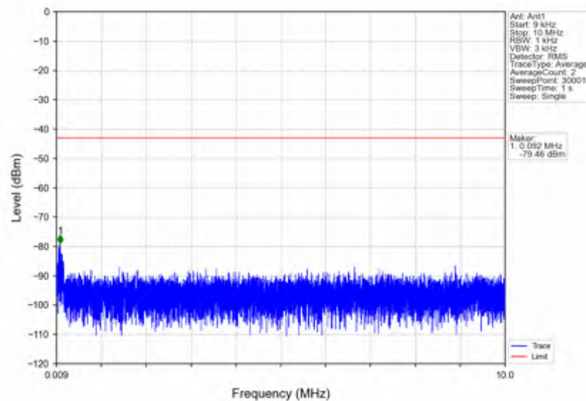
n7_15kHz_SISO_NTNV_20MHz_DFT-s-OFDM QPSK_2510MHz_Inner_1RB_Left
