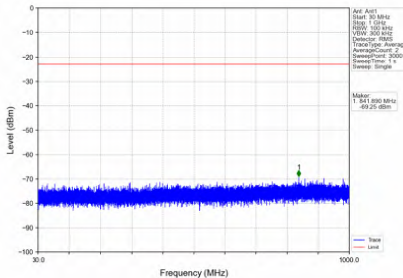
n7_15kHz_SISO_NTNV_20MHz_CP-OFDM QPSK_2535MHz_Edge_1RB_Left
