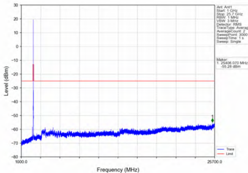
n7_15kHz_SISO_NTNV_20MHz_CP-OFDM QPSK_2535MHz_Edge_1RB_Left
