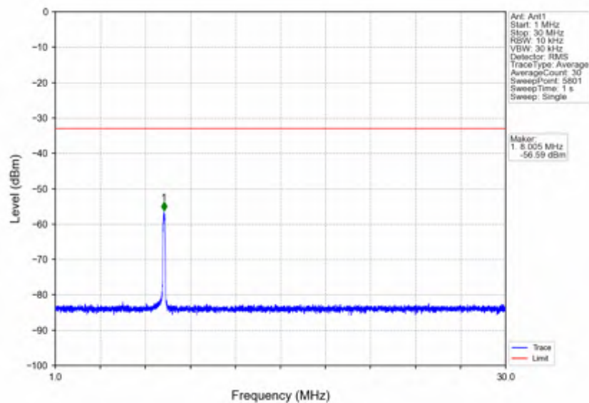
n7 15kHz SISO NTN 20MHz DFT-s-OFDM QPSK 2560MHz Inner 1RB Right
