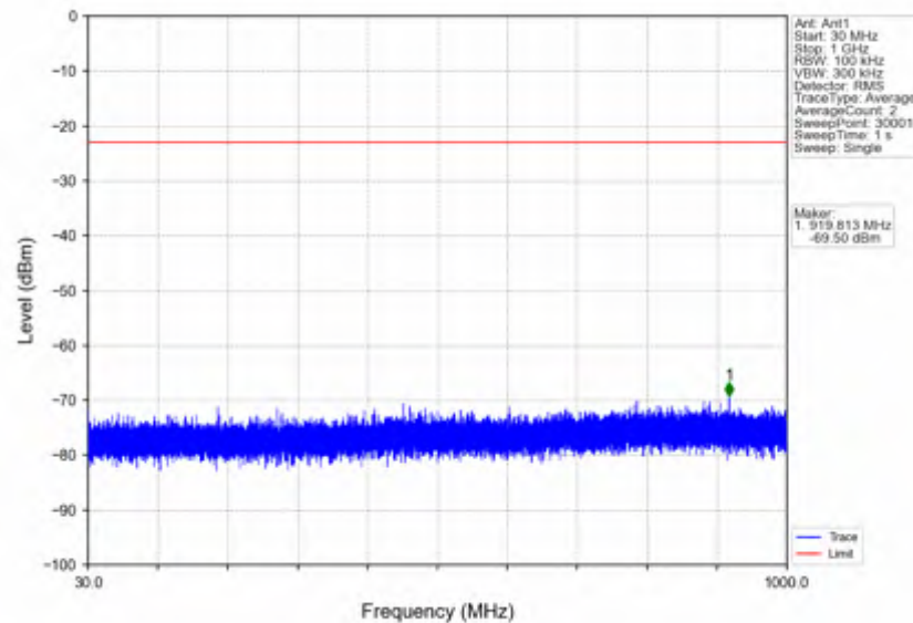
n7_15kHz_SISO_NTNV_10MHz_DFT-s-OFDM PI/2 BPSK_2505MHz_Inner_1RB_Left
