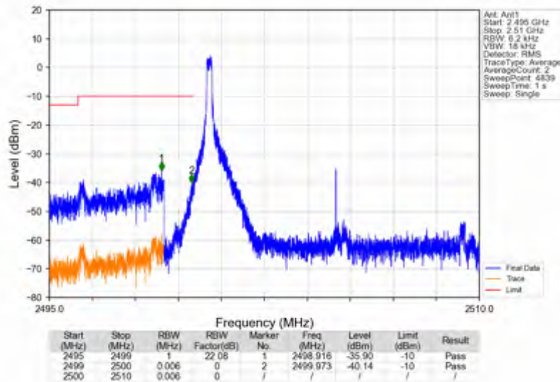
n7_15kHz_SISO_NTNV_10MHz_CP-OFDM_QPSK_2505MHz_Inner_1RB_Left
