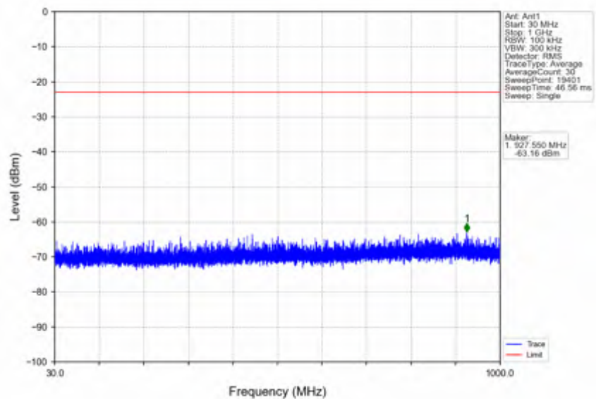
n38_30kHz_SISO_NTNV_30MHz_DFT-s-OFDM PI/2 BPSK_2585MHz_Edge_1RB_Left
