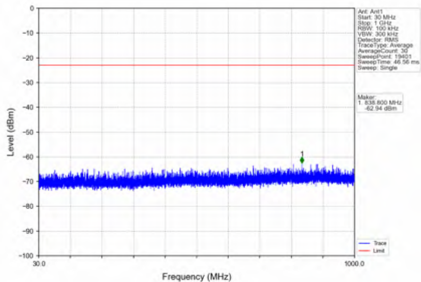
n38_30kHz_SISO_NTNV_30MHz_CP-OFDM QPSK_2595MHz_Edge_1RB_Left
