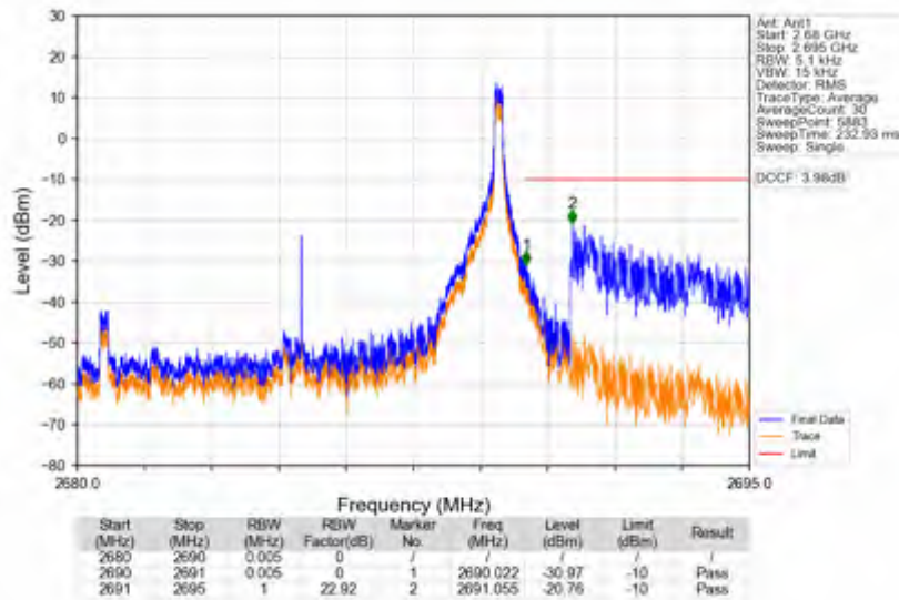
n41_15kHz_SISO_NTNV_10MHz_DFT-s-OFDM QPSK_2685MHz_Inner_1RB_Right
