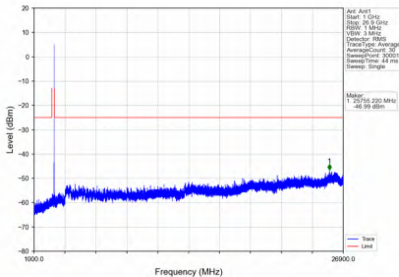
n41_15kHz_SISO_NTNV_10MHz_DFT-s-OFDM QPSK 2501.01MHz_Edge_1RB_Left
