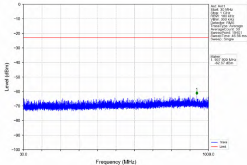
n38_30kHz_SISO_NTNV_40MHz_DFT-s-OFDM QPSK_2595MHz_Edge_1RB_Left
