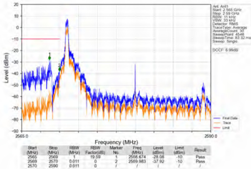
n38_30kHz_SISO_NTNV_20MHz_DFT-s-OFDM_QPSK_2580MHz_Edge_1RB_Left
