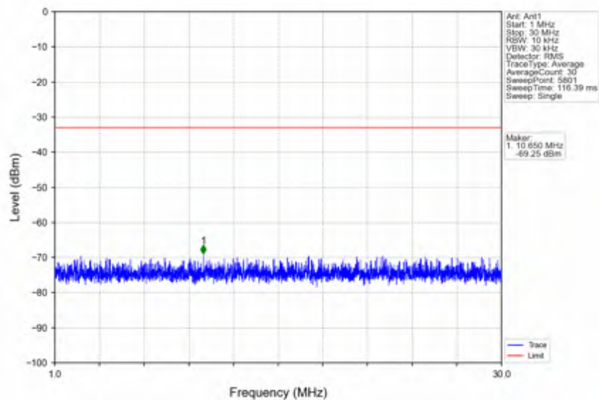
n41_15kHz_SISO_NTNV_10MHz_DFT-s-OFDM QPSK_2501.01MHz_Edge_1RB_Left
