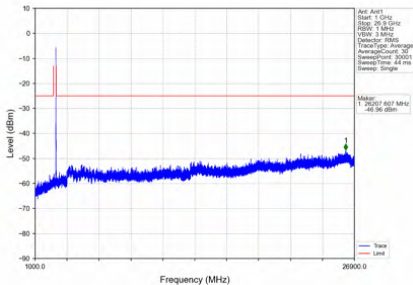
n41_15kHz_SISO_NTNV_10MHz_DFT-s-OFDM QPSK_2685MHz_Inner_1RB_Right
