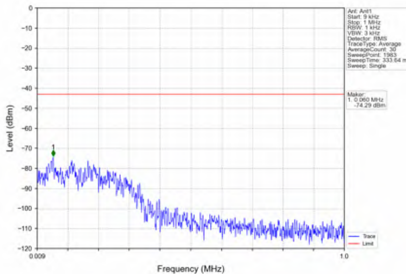
n38 30kHz SISO NTN 25MHz CP-OFDM QPSK 2595MHz Edge 1RB Left
