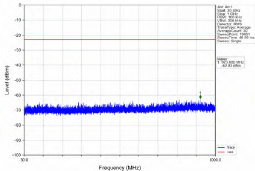
n38 30kHz SISO NTN 30MHz CP-OFDM QPSK 2605MHz Edge 1RB Right
