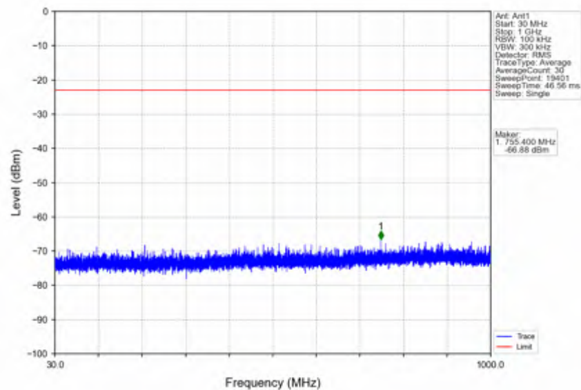
n41_15kHz_SISO_NTNV_10MHz_DFT-s-OFDM PI/2 BPSK_2685MHz_Inner_1RB_Right
