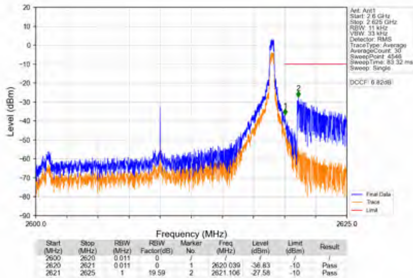
n38 30kHz SISO NTN 20MHz CP-OFDM QPSK 2610MHz Edge 1RB Right
