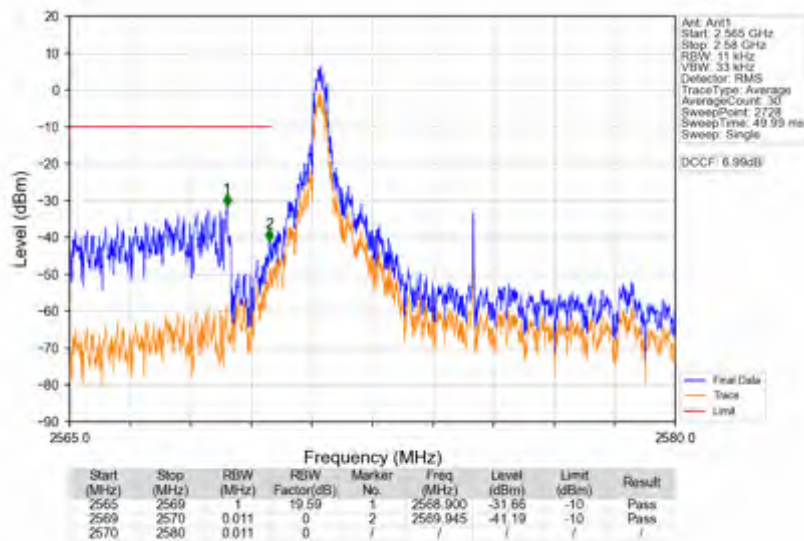
n38_30kHz_SISO_NTNV_10MHz_CP-OFDM QPSK_2575MHz_Inner_1RB_Left
