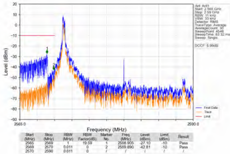
n38_30kHz_SISO_NTNV_20MHz_DFT-s-OFDM PI/2 BPSK_2580MHz_Inner_1RB_Left
