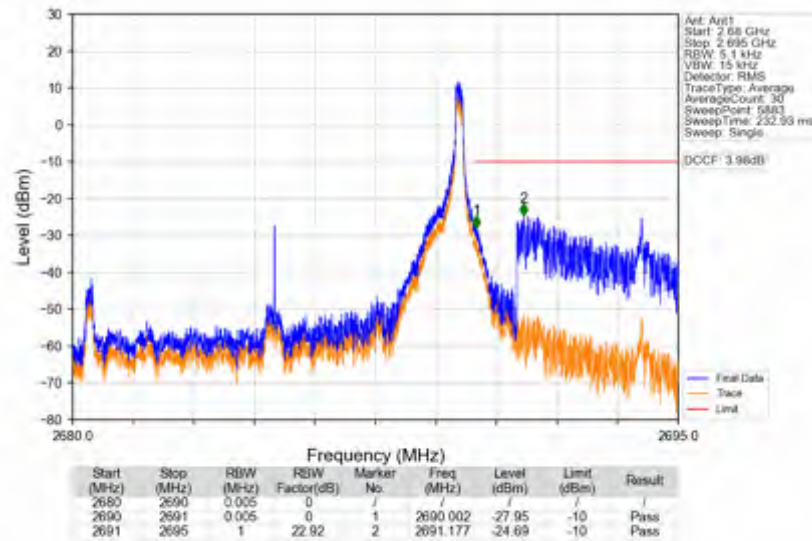
n41_15kHz_SISO_NTNV_10MHz_DFT-s-OFDM PI/2 BPSK_2685MHz_Edge_1RB_Right
