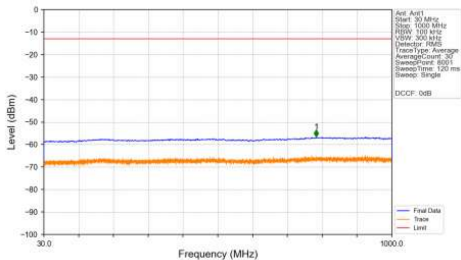
n66_15kHz_SISO_NTNV_20MHz_DFT-s-OFDM_QPSK_1720MHz_Edge_1RB_Left_Ant1
