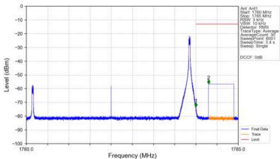
n66_15kHz_SISO_NTNV_20MHz_DFT-s-OFDM_QPSK_1770MHz_Inner_1RB_Right_Ant1
