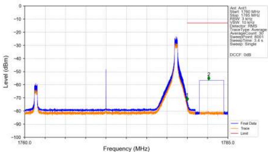
n66_30kHz_SISO_NTNV_20MHz_CP-OFDM_QPSK_1770MHz_Inner_1RB_Right_Ant1
