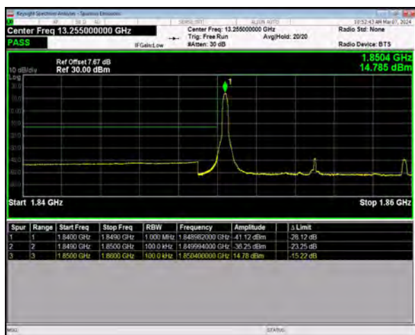
n25 SCS=15kHz DFT_256QAM BW=10MHz
