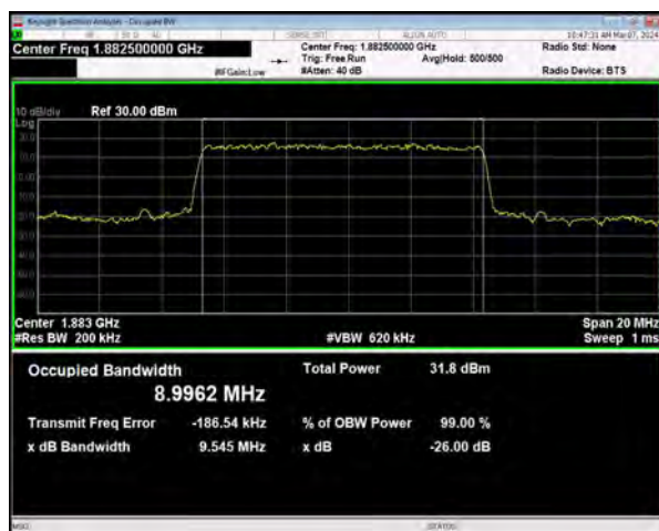
n25 SCS=15kHz DFT_BPSK BW=10MHz Channel=376500 RB=50@0
