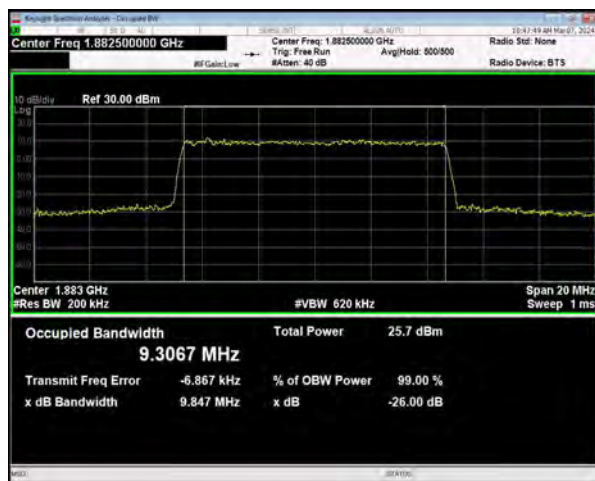
n25 SCS=15kHz CP_256QAM BW=10MHz Channel=376500 RB=52@0
