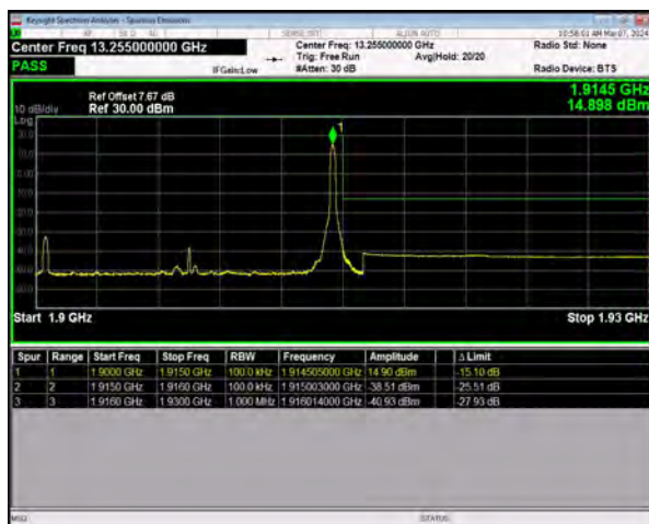
n25 SCS=15kHz DFT_256QAM BW=15MHz
