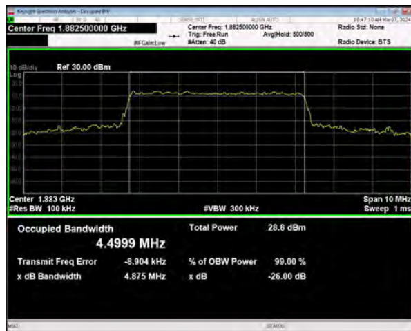
n25 SCS=15kHz CP_QPSK BW=5MHz Channel=376500 RB=25@0
