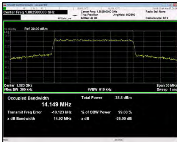
n25 SCS=15kHz CP_64QAM BW=15MHz Channel=376500 RB=79@0
