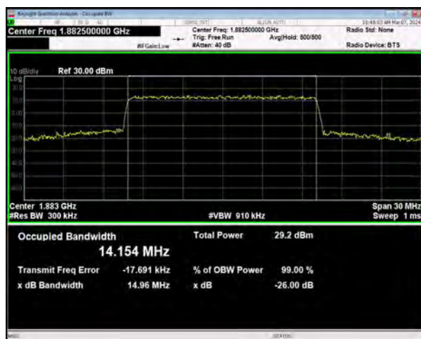
n25 SCS=15kHz CP_QPSK BW=15MHz Channel=376500 RB=79@0
