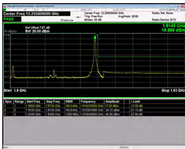
n25 SCS=15kHz DFT_64QAM BW=15MHz
