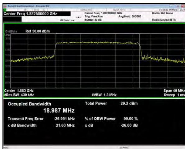
n25 SCS=15kHz CP_16QAM BW=20MHz Channel=376500 RB=106@0
