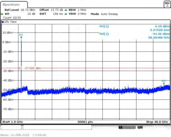
11AX80MIMO_Ant1_5610_1000~40000
