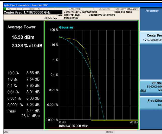
Band4-1.4MHz-QPSK-19957-1-0-Low-7.95-&lt;=13-PASS
