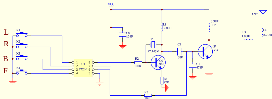
电子板HX-PB068T-8(JZ)发射原理图
