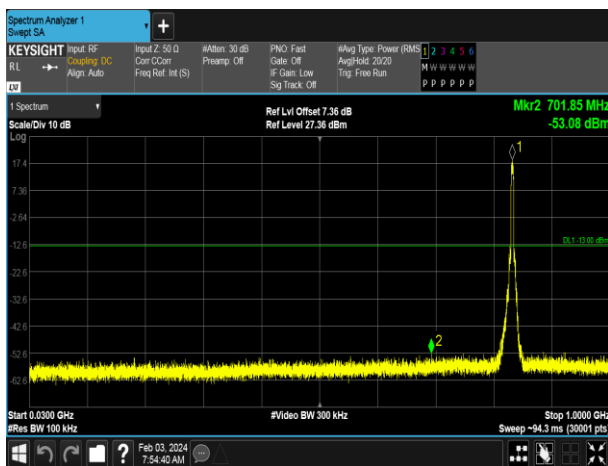
WCDMA 850 RMC 12.2kps HCH
