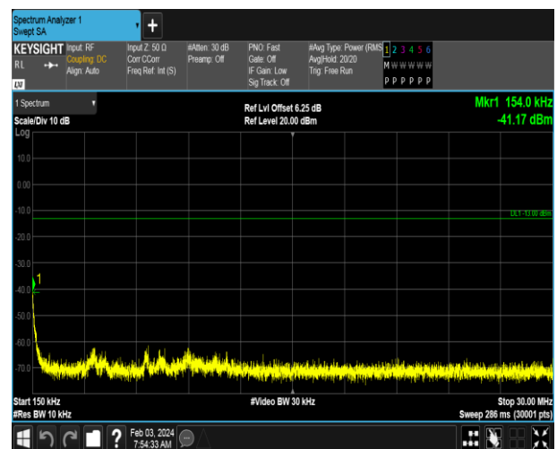
WCDMA 850 RMC 12.2kps HCH
