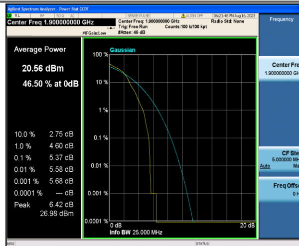
Band2-20MHz-16QAM-19100-1RB#0-PASS
