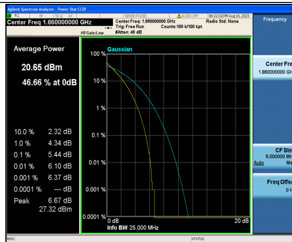
Band2-20MHz-QPSK-18700-100RB#0-PASS
