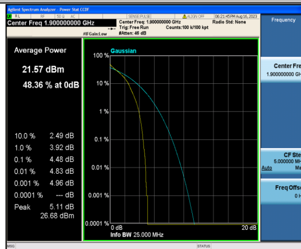
Band2-20MHz-QPSK-19100-1RB#0-PASS
