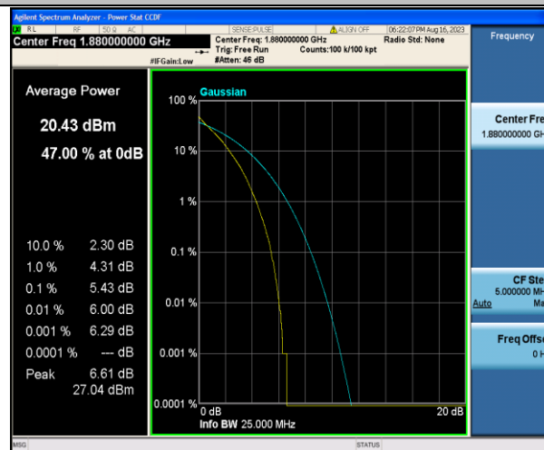
Band2-20MHz-QPSK-18900-100RB#0-PASS
