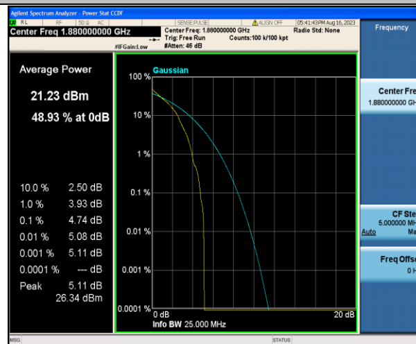
Band2-5MHz-QPSK-18900-1RB#0-PASS
