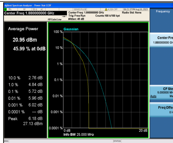
Band2-20MHz-16QAM-18900-1RB#0-PASS
