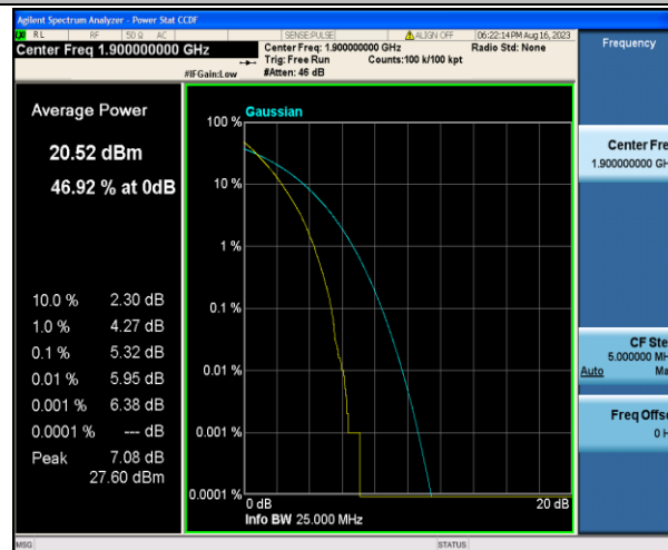
Band2-20MHz-QPSK-19100-100RB#0-PASS
