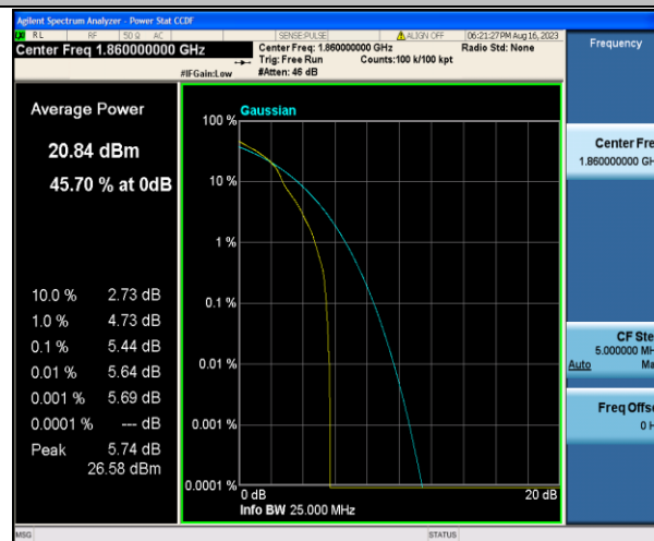
Band2-20MHz-16QAM-18700-1RB#0-PASS
