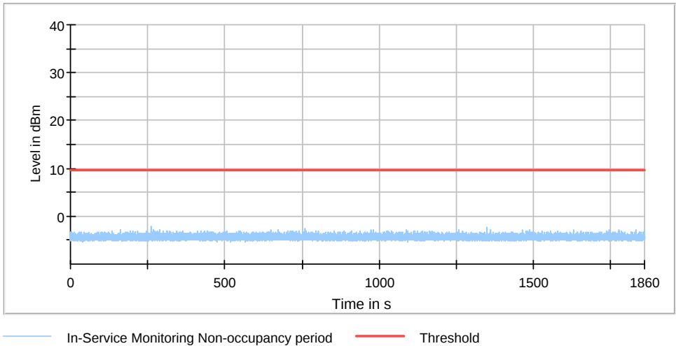
IEEE 802.11ac VHT80 5530MHz
