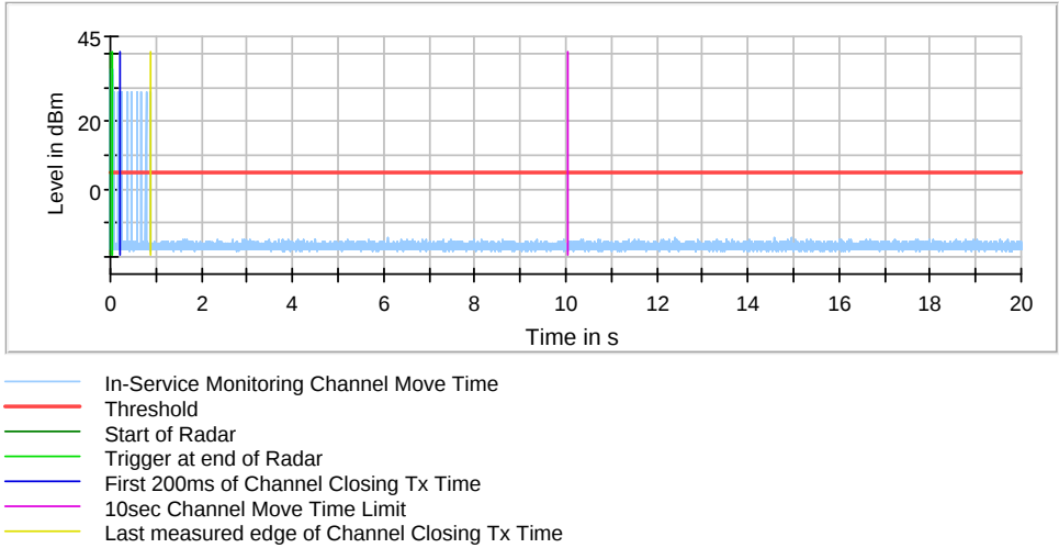
IEEE 802.11a 5500MHz
