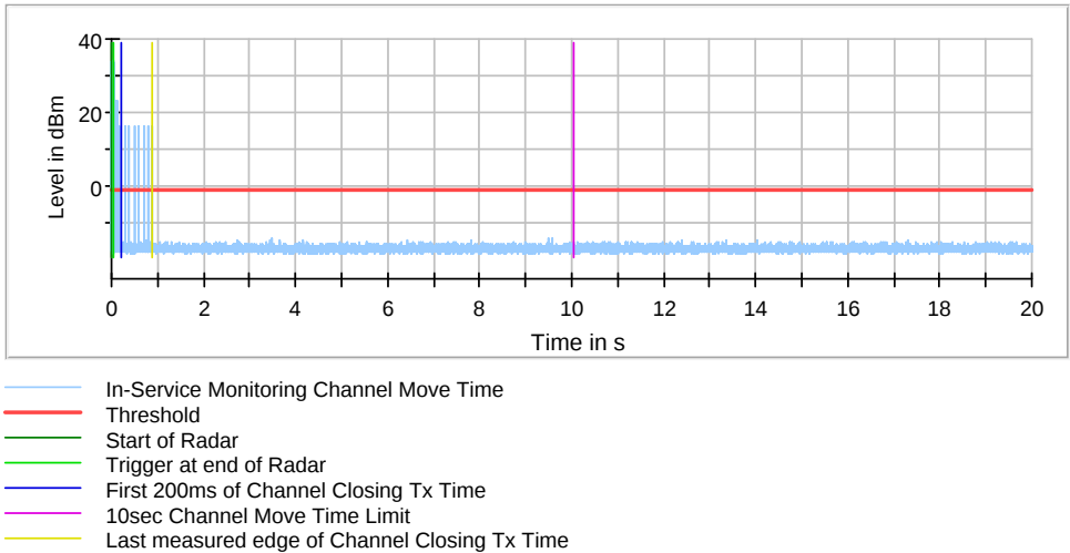
IEEE 802.11n HT40 5510MHz
