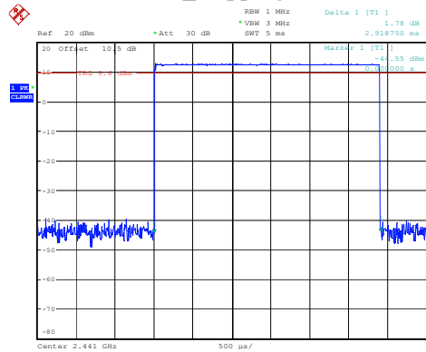
DH5_Hopping 2.919ms
