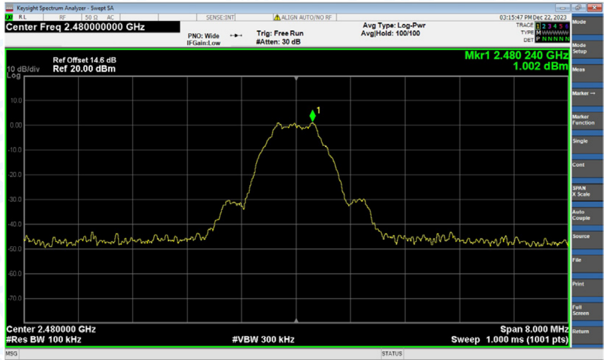
Band Edge NVNT BLE 1Mbps 2480MHz Ant1 Emission
