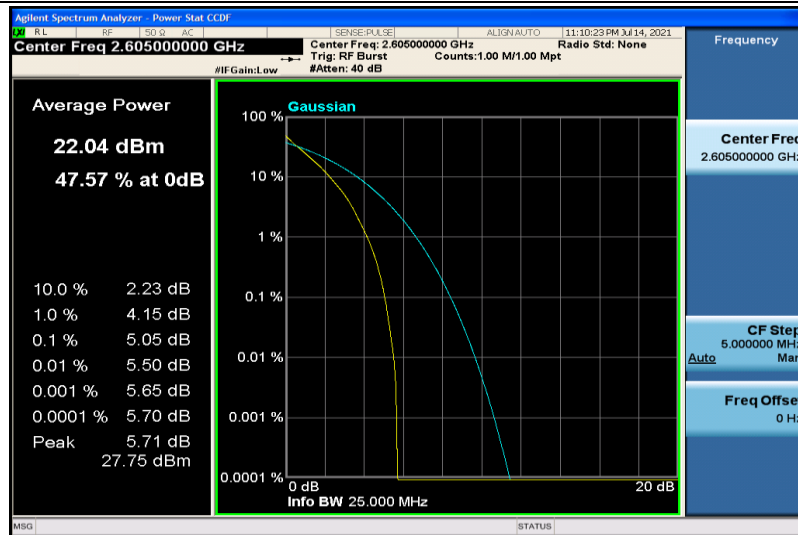
Band41-10MHz-QPSK-40740-50RB#0
