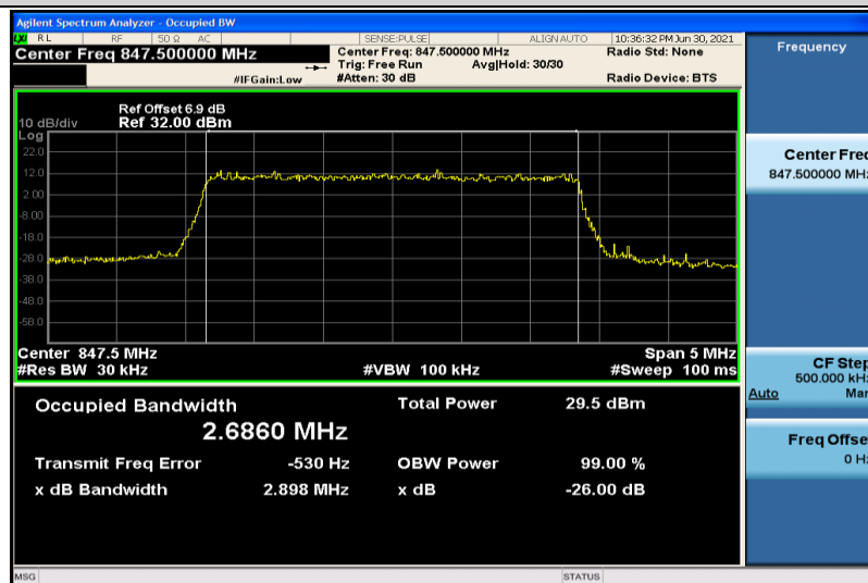
Band5-3MHz-QPSK-20635-15RB#0-2.6860
