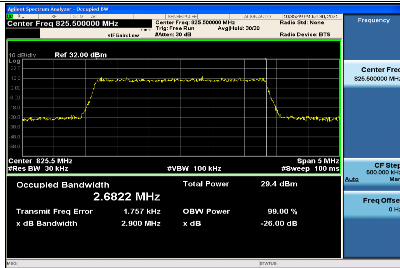
Band5-3MHz-QPSK-20415-15RB#0-2.6822
