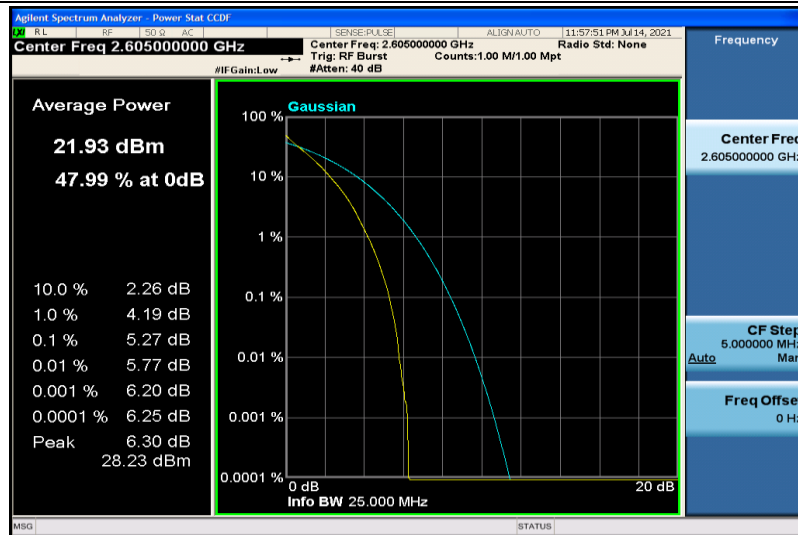
Band41-20MHz-QPSK-40740-100RB#0
