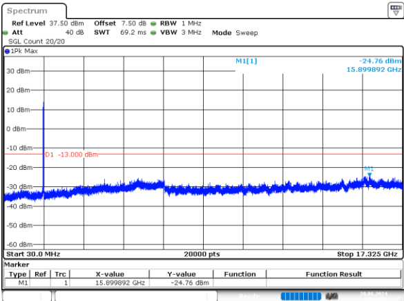
20MHz_Middle_QPSK_100@0 -24.76dBm
