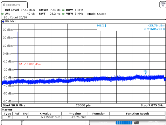
1.4MHz_Middle_QPSK_1@0 -25.76dBm
