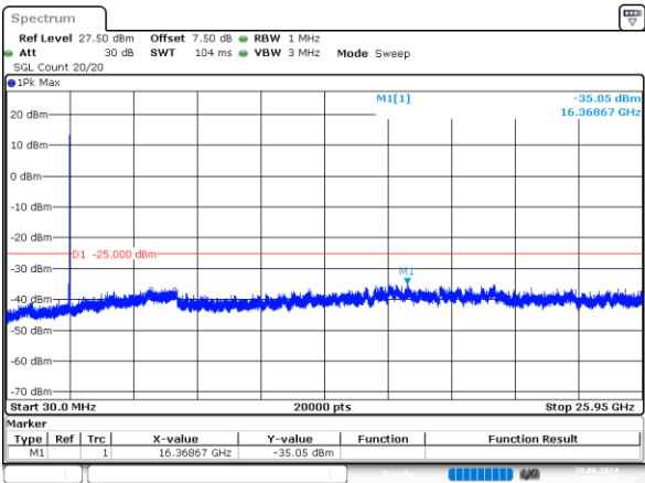
5MHz_Middle_QPSK_25@0 -35.05dBm
