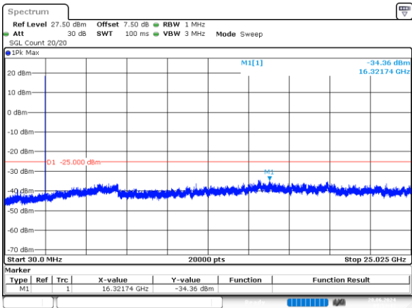
5MHz_Low_QPSK_1@0 -34.36dBm
