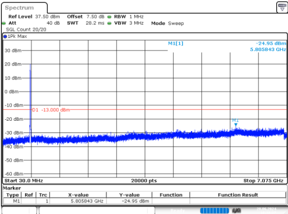
10MHz_Middle_QPSK_50@0 -24.95dBm
