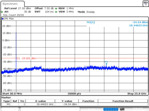
20MHz_Low_QPSK_100@0 -34.54dBm
