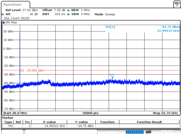
10MHz_Low_QPSK_1@0 -34.75dBm
