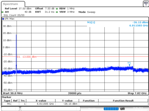
10MHz_Middle_QPSK_50@0 -26.15dBm
