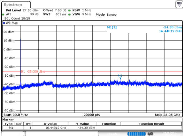
10MHz_Low_QPSK_50@0 -34.30dBm
