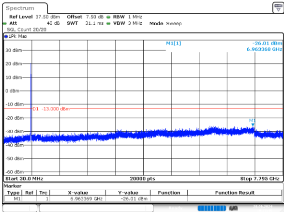
5MHz_Low_QPSK_25@0 -26.01dBm
