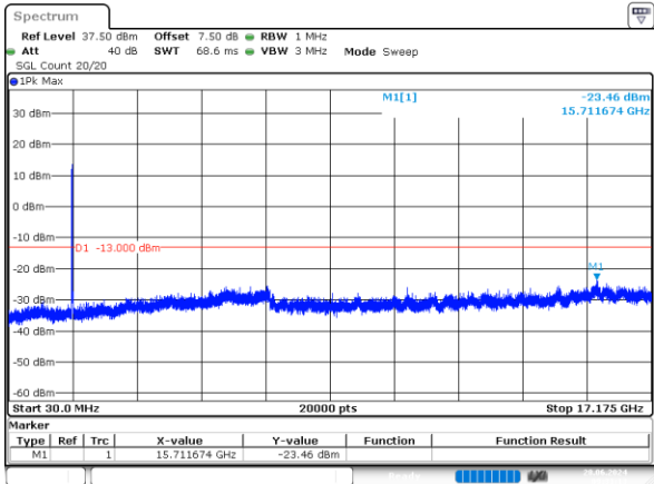
15MHz_Low_QPSK_75@0 -23.46dBm
