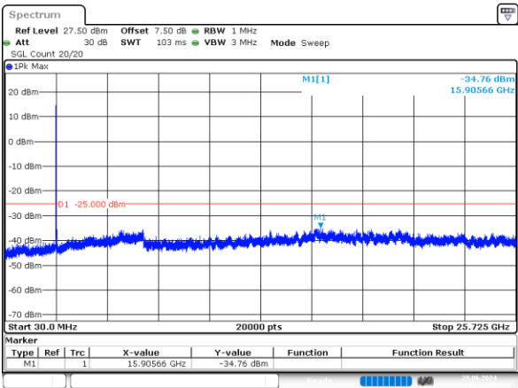
5MHz_Low_QPSK_25@0 -34.76dBm
