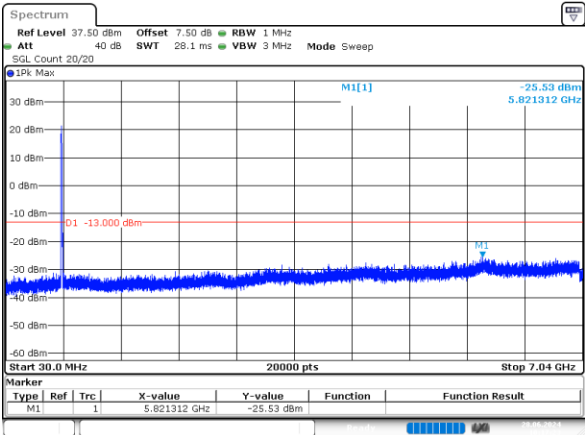
10MHz_Low_QPSK_50@0 -25.53dBm
