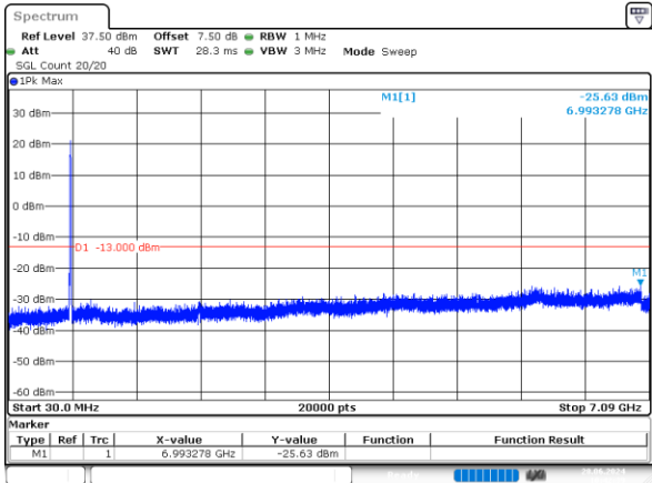
10MHz_Low_QPSK_50@0 -25.63dBm
