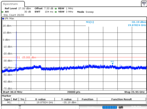
10MHz_Middle_QPSK_50@0 -35.19dBm
