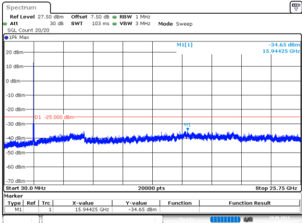
10MHz_Low_QPSK_50@0 -34.65dBm
