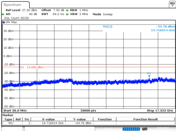
15MHz_Middle_QPSK_75@0 -24.76dBm
