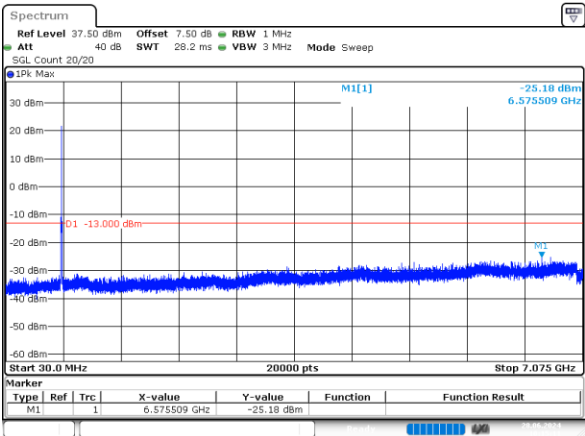
5MHz_Middle_QPSK_25@0 -25.18dBm
