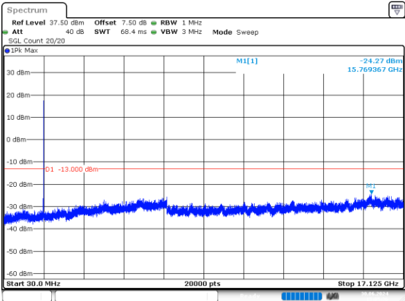
5MHz_Low_QPSK_25@0 -24.27dBm
