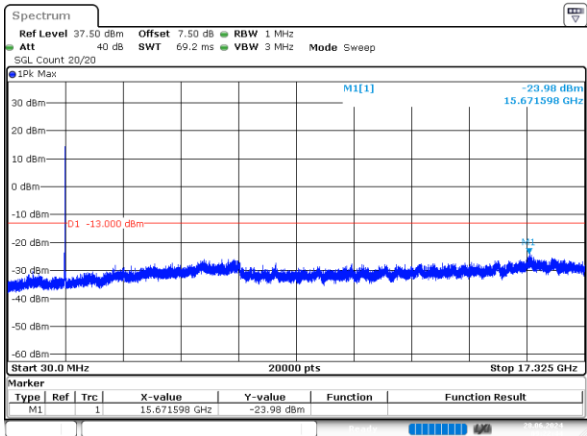
10MHz_Middle_QPSK_50@0 -23.98dBm
