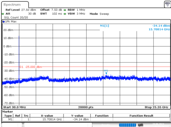
10MHz_Middle_QPSK_50@0 -34.14dBm
