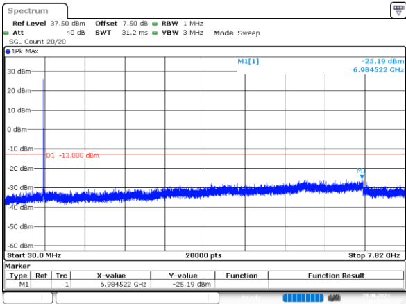
10MHz_Middle_QPSK_1@0 -25.19dBm
