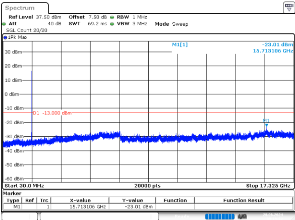
5MHz_Middle_QPSK_25@0 -23.01dBm
