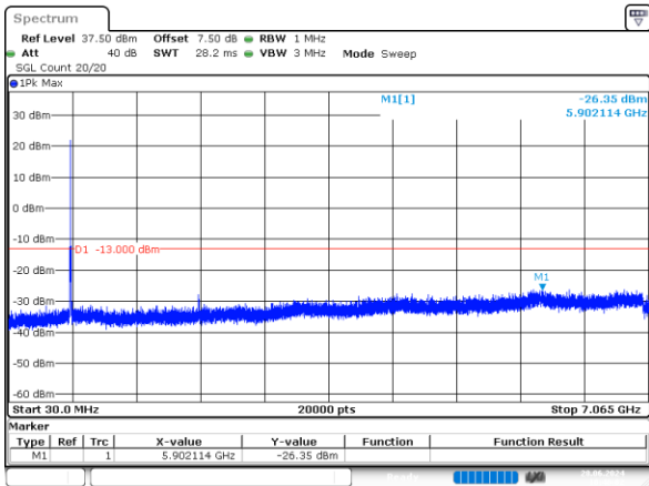
5MHz_Low_QPSK_25@0 -26.35dBm
