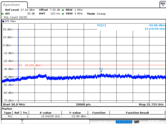
5MHz_Low_QPSK_1@0 -33.88dBm
