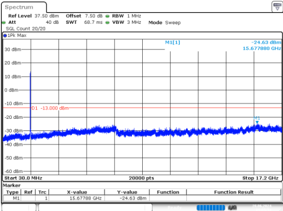
20MHz_Low_QPSK_100@0 -24.63dBm
