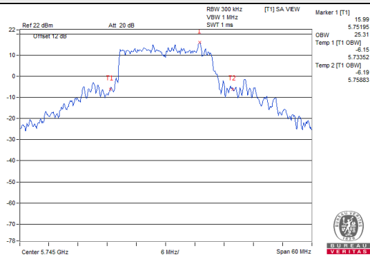
802.11ax (20MHz) / Chain 2 / CH 149
