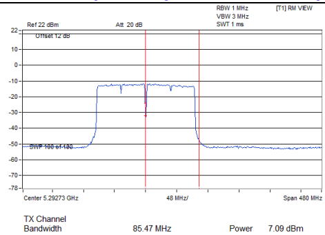
802.11ac (160MHz)_Chain 0: CH 50(For U-NII-2A)
