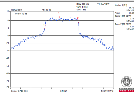
802.11ax (20MHz) / Chain 3 / CH 149
