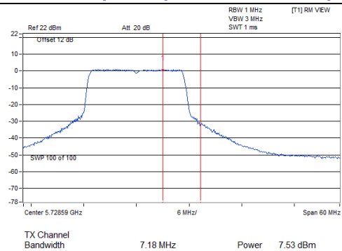
802.11an (20MHz)_Chain 1: CH 144(For U-NII-3)
