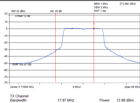
802.11an (20MHz)_Chain 0: CH 144 (For U-NII-2C)
