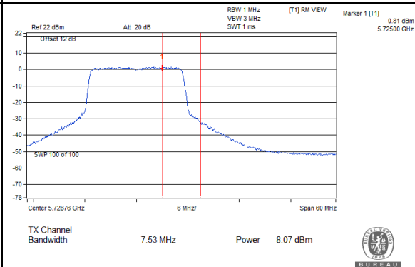
802.11ac (20MHz)_Chain 3: CH 144(For U-NII-3)
