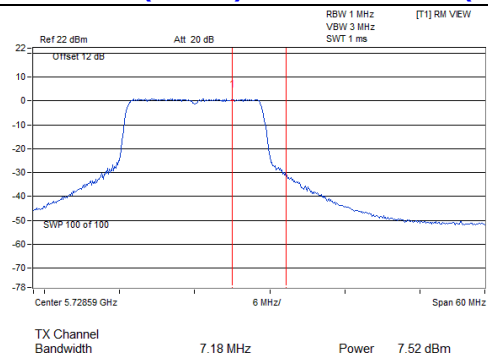
802.11an (20MHz)_Chain 2: CH 144(For U-NII-3)
