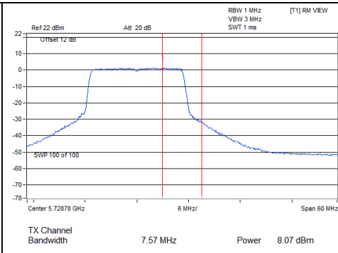
802.11ac (20MHz)_Chain 3: CH 144(For U-NII-3)
