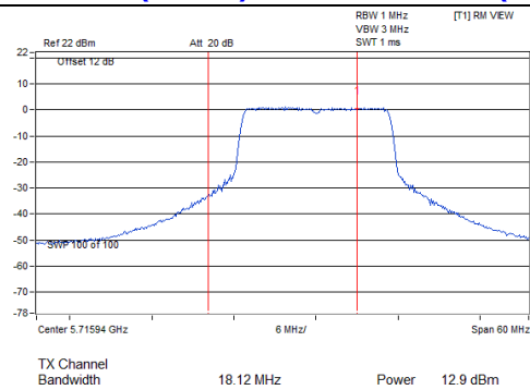
802.11an (20MHz)_Chain 2: CH 144 (For U-NII-2C)
