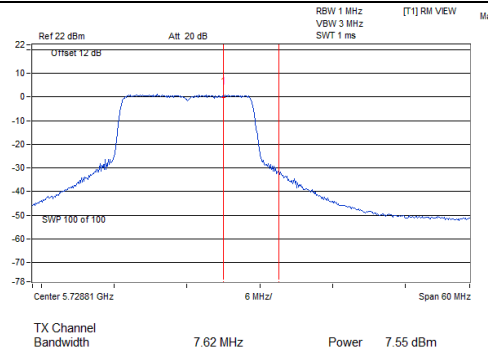
802.11an (20MHz)_Chain 0: CH 144(For U-NII-3)
