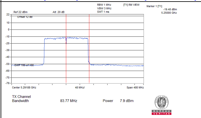
802.11ax (160MHz)_Chain 3: CH 50(For U-NII-2A)
