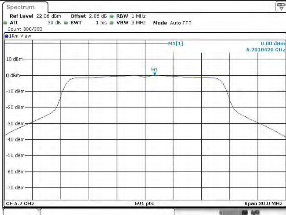
11A_Ant1_5700
