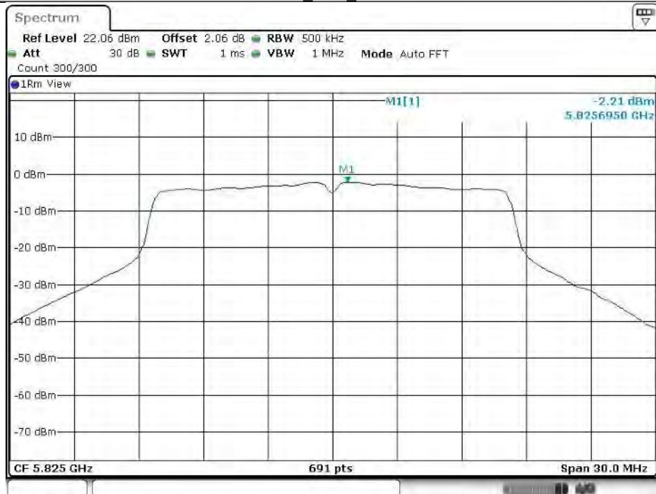
11A_Ant2_5825
