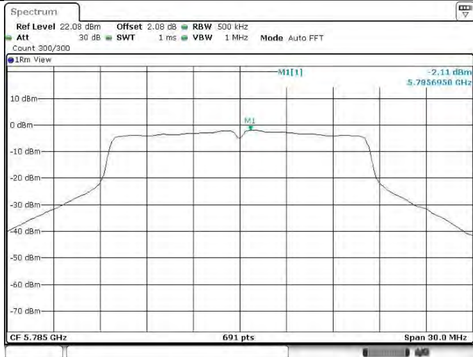
11A_Ant2_5785
