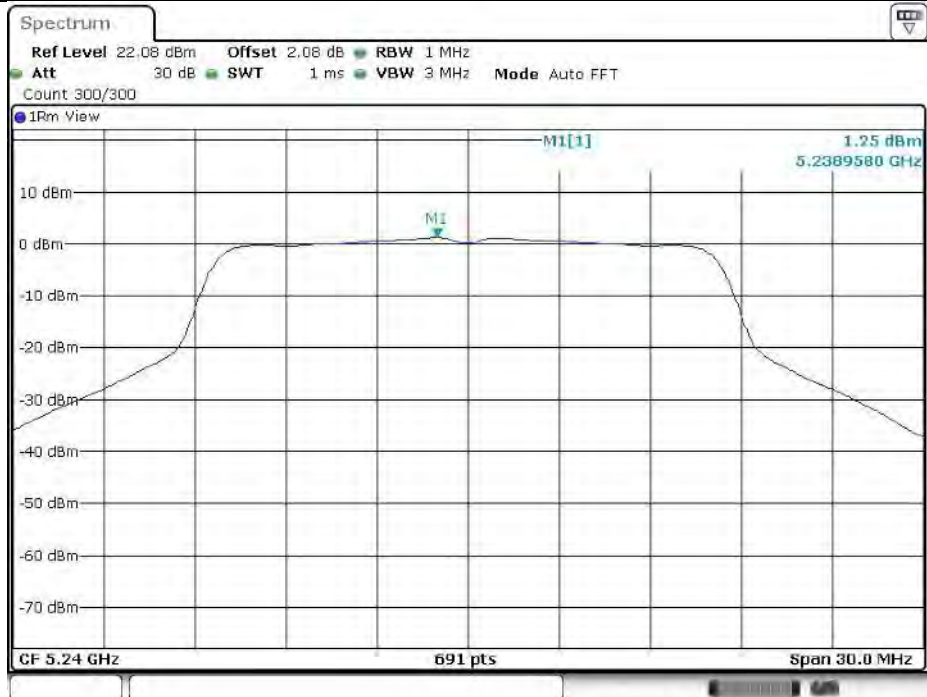
11A_Ant2_5240
