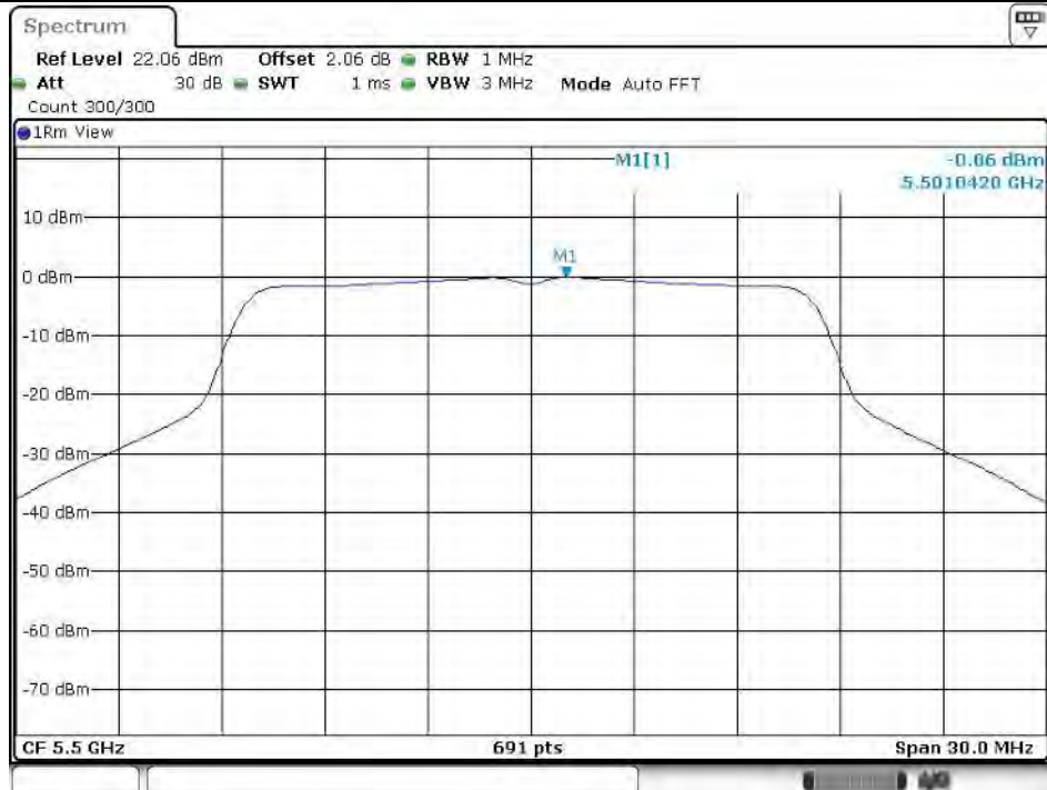
11A_Ant1_5500
