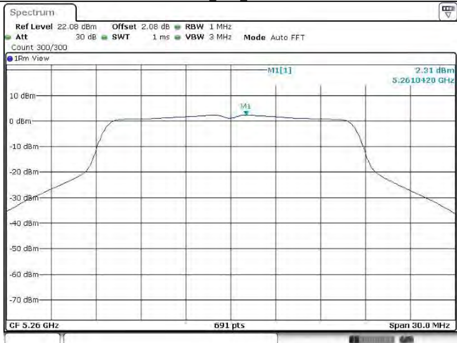
11A_Ant1_5260
