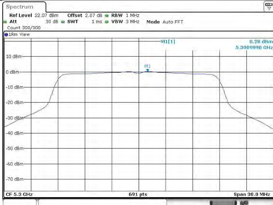
11N20SISO_Ant2_5300
