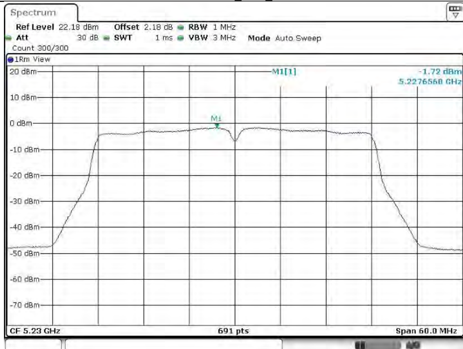
11N40SISO_Ant2_5230
