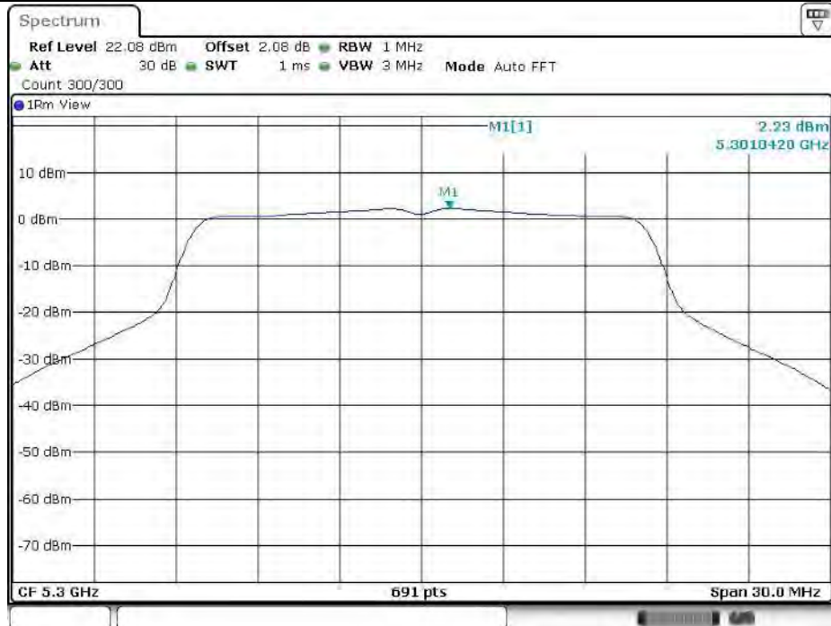
11A_Ant1_5300
