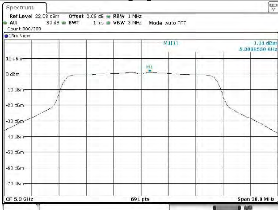
11A_Ant2_5300
