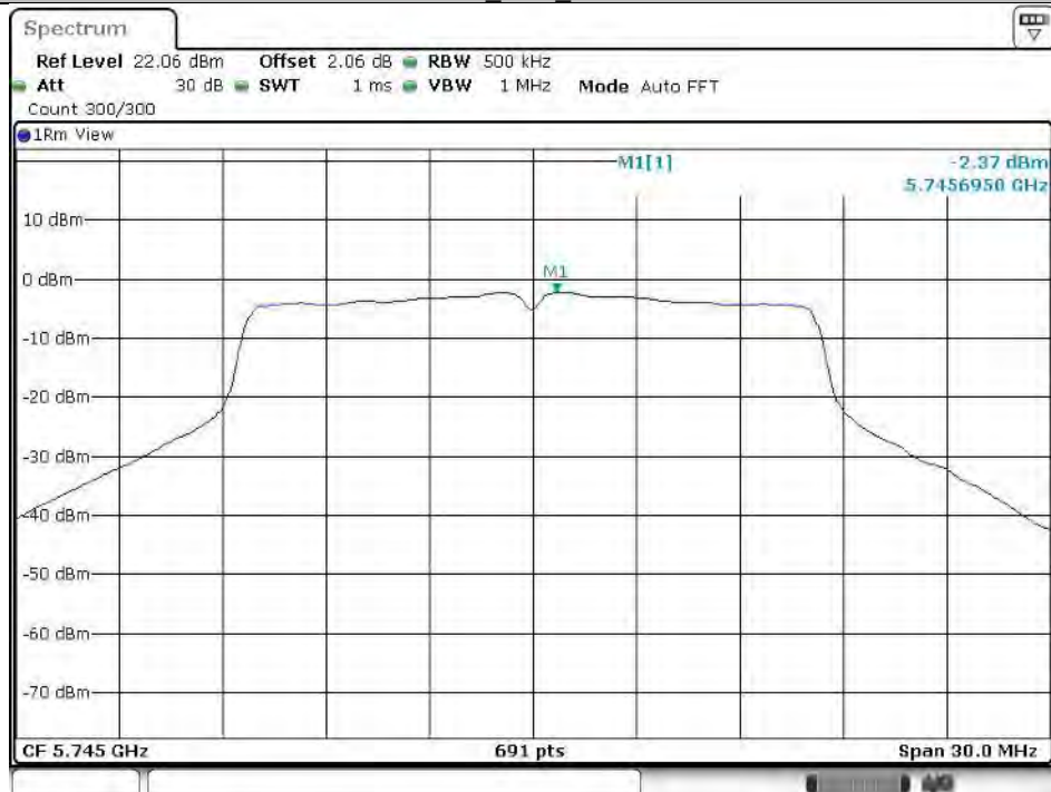
11A_Ant2_5745
