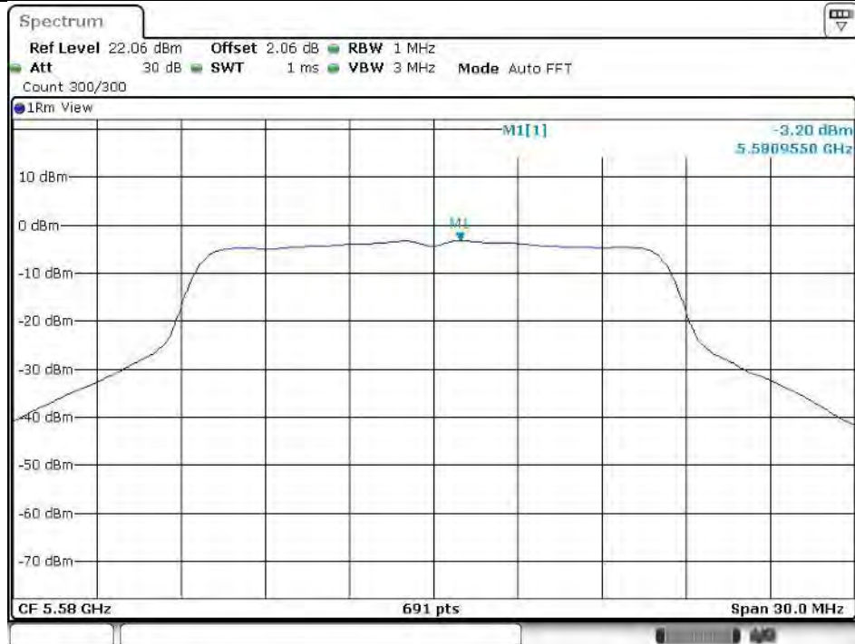
11A_Ant2_5580
