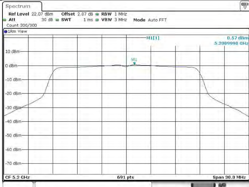
11N20SISO_Ant2_5200
