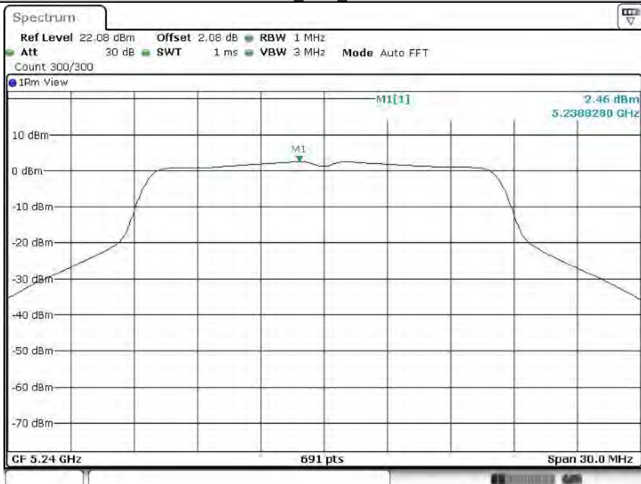
11A_Ant1_5240
