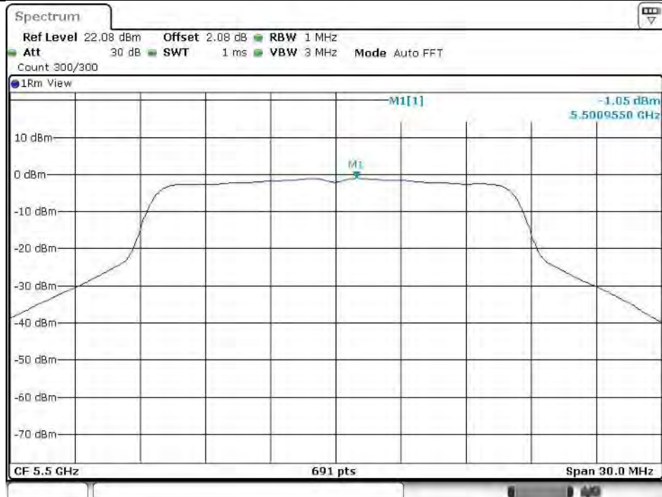
11A_Ant2_5500
