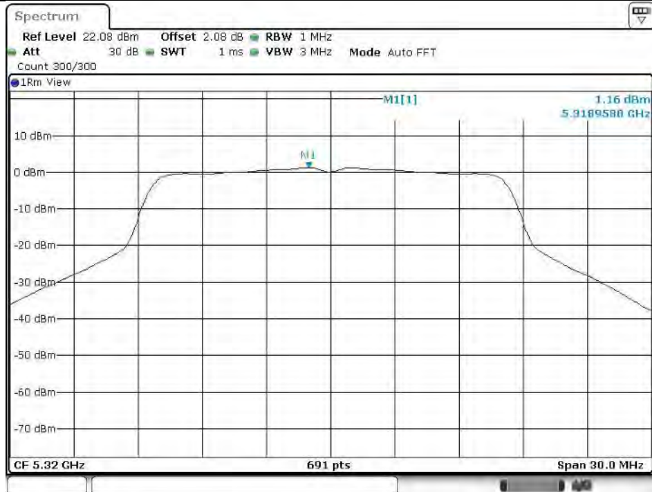
11A_Ant2_5320
