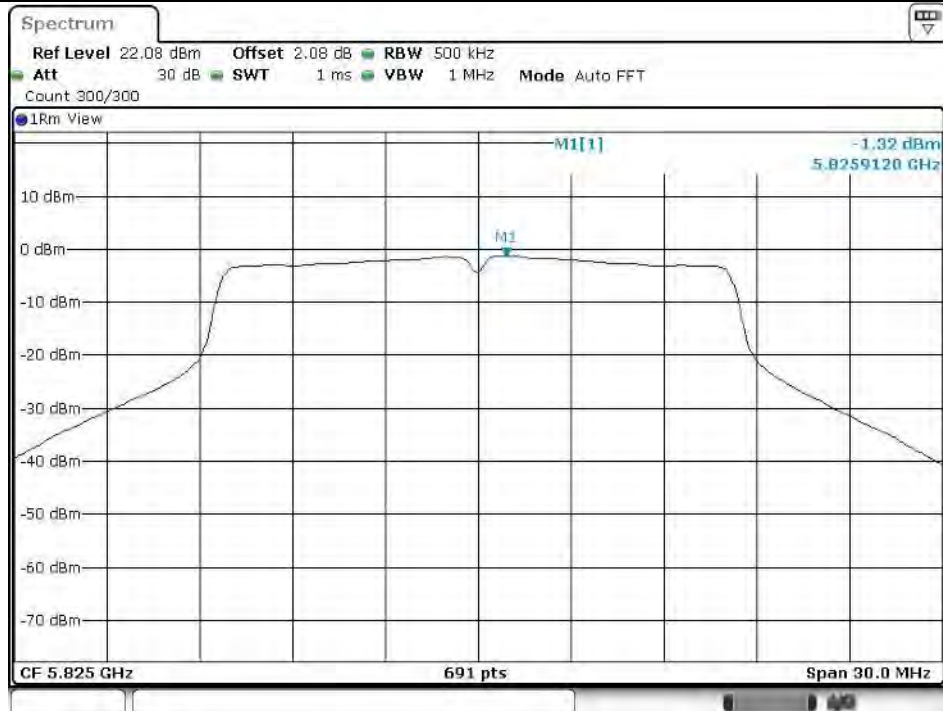
11A_Ant1_5825
