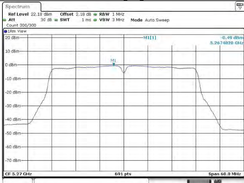
11N40SISO_Ant1_5270
