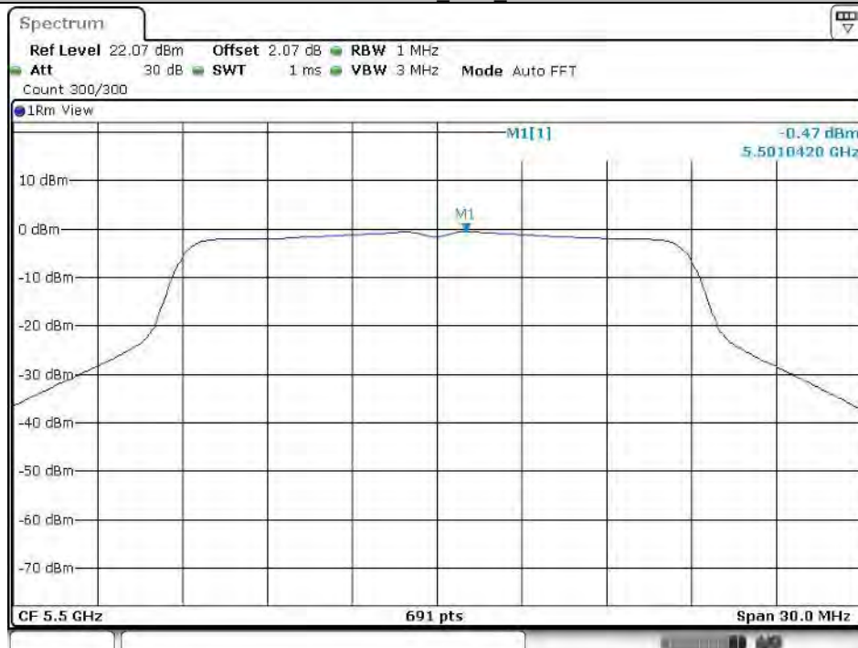
11N20SISO_Ant1_5500
