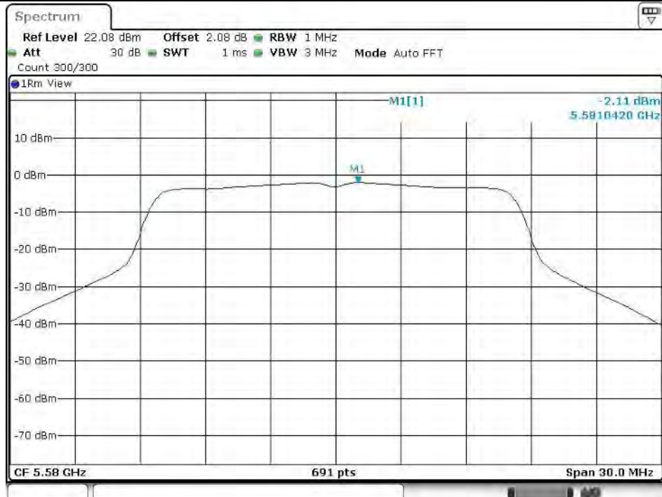
11A_Ant1_5580
