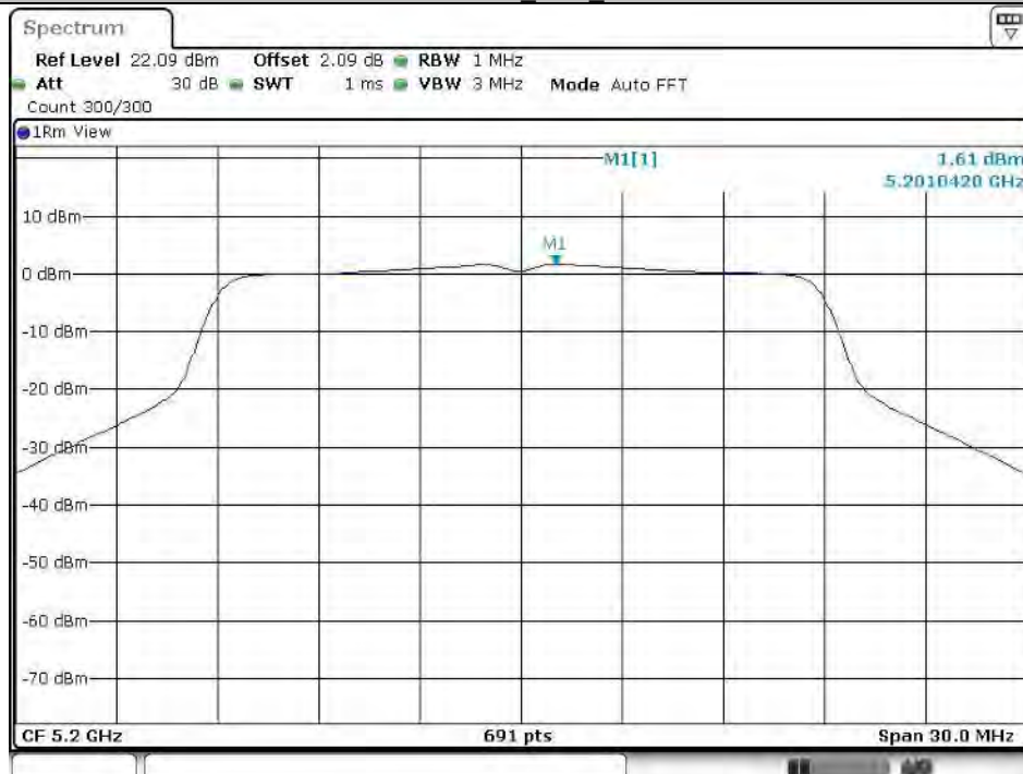
11N20SISO_Ant1_5200
