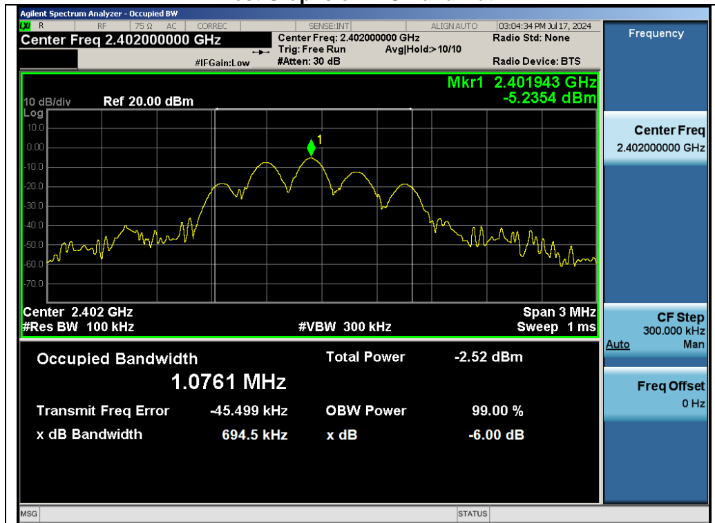
Test_Graph_ANT1_2402_DTBSW
