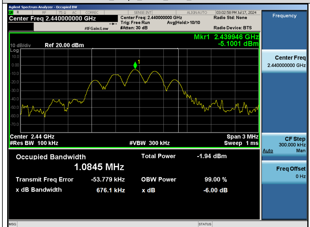
Test_Graph_ANT1_2440_DTBSW
