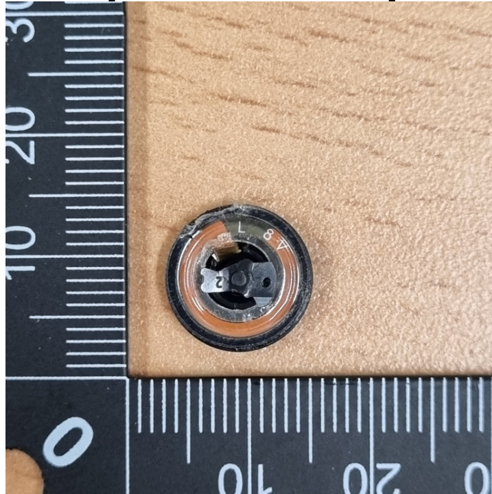
[Earbud_Left_Antenna]
