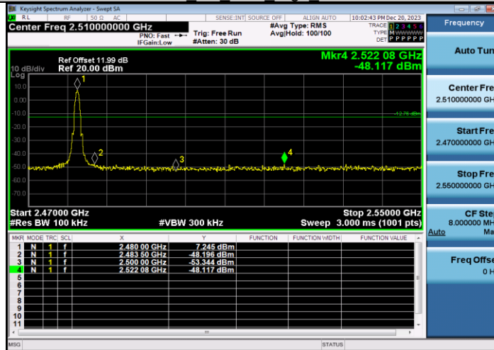
BLE 1M Ant1 High 2480
