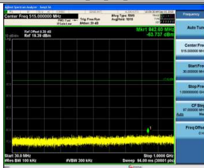
11G-CDD_Ant2_2422_30~1000
