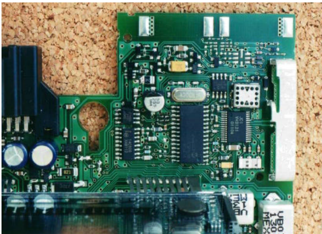
FN145-DB RF Section - Top
