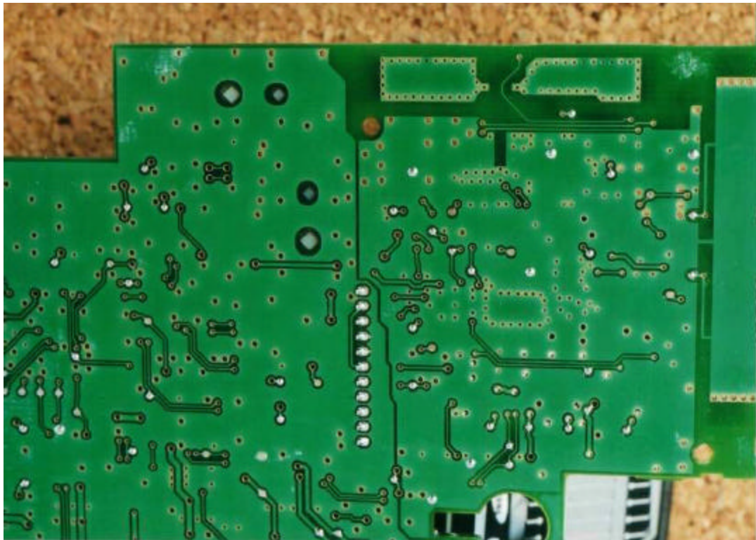
FN145-JB RF Section - Bottom
