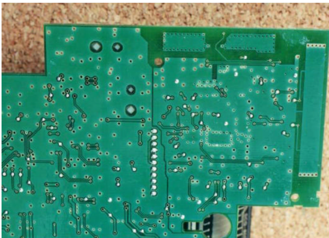
FN145-DB RF Section - Bottom
