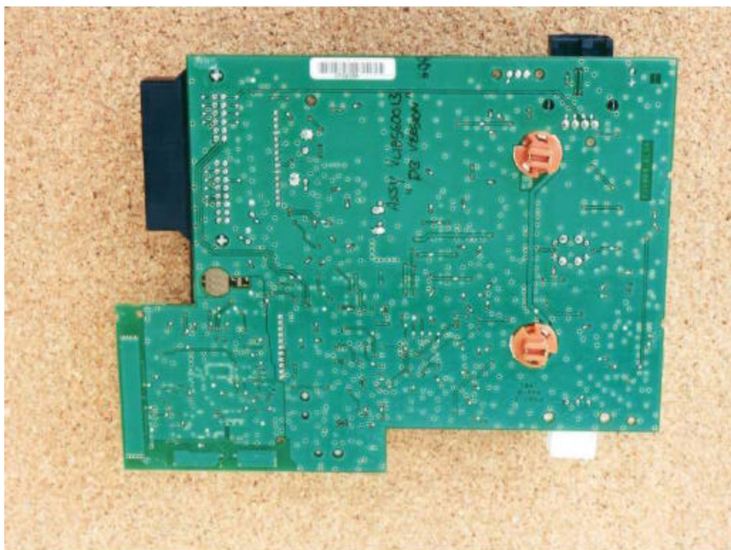
FN145-DB PCB - Bottom
