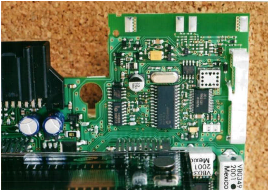
FN145-JB RF Section - Top
