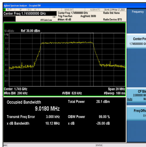
Band66-10MHz-QPSK-132322-50RB#0-9.0180
