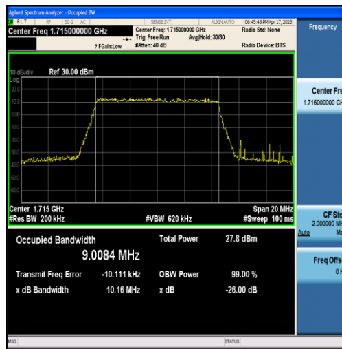
Band66-10MHz-QPSK-132022-50RB#0-9.0084
