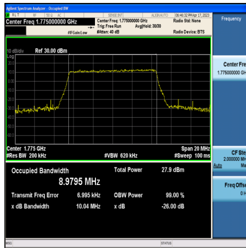
Band66-10MHz-QPSK-132622-50RB#0-8.9795
