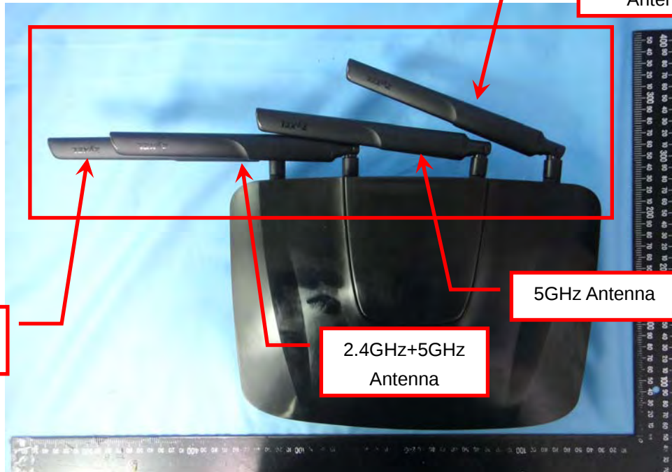
EUT Photo 1 )
