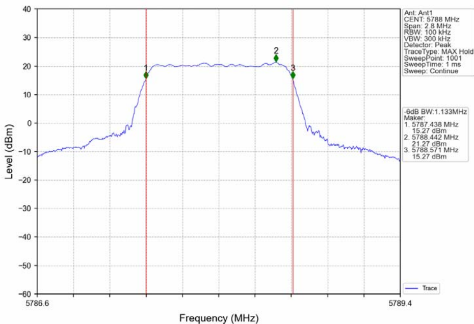
QPSK 1.4MHz_MCH_5788MHz_Ant1_NTNV
