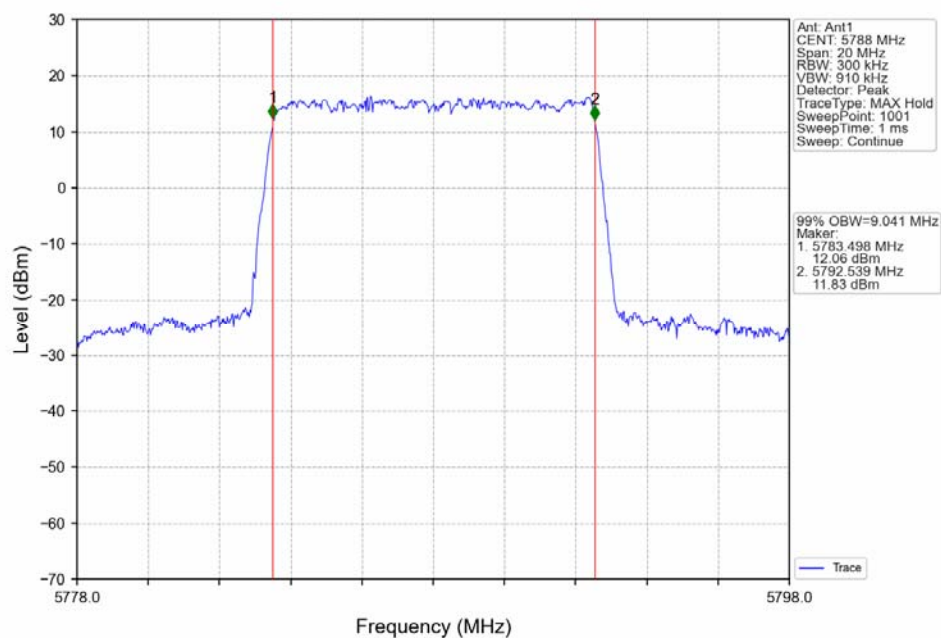
QPSK 10MHz_MCH_5788MHz_Ant1_NTNV
