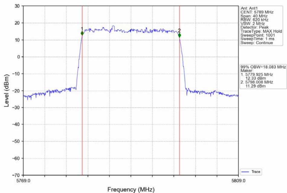
QPSK 20MHz_MCH_5789MHz_Ant1_NTNV
