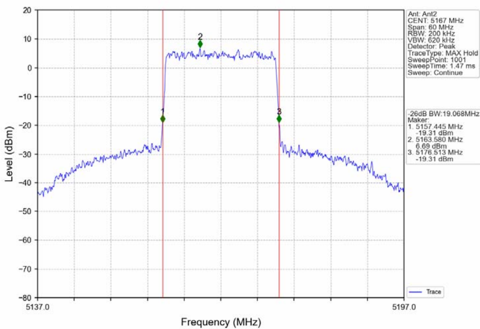
QPSK 20MHz_LCH_5167MHz_Ant2_NTNV
