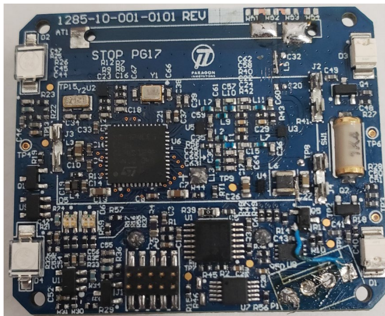
Top of BLUBand V3 PCB
