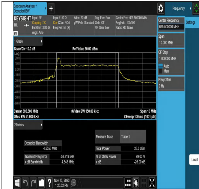
NTVN_N71_PC3_15_5_H_TID5_Ant1#1
