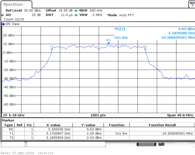
11AX20MIMO-Ant1-5180
