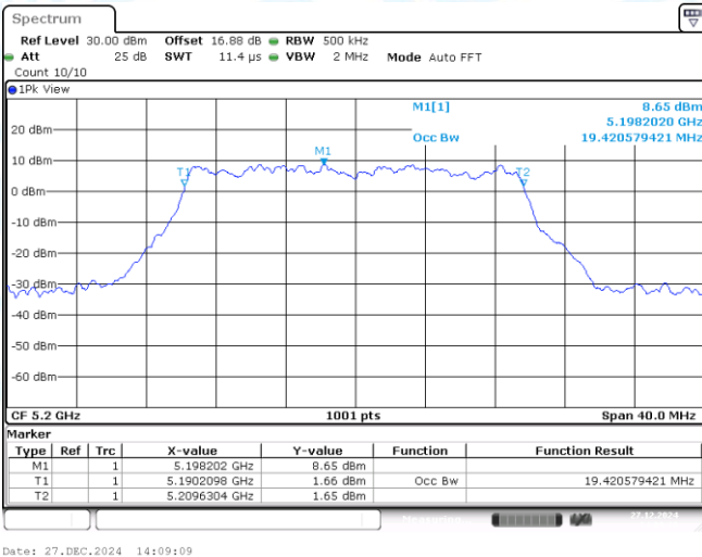
11AX20MIMO-Ant1-5200
