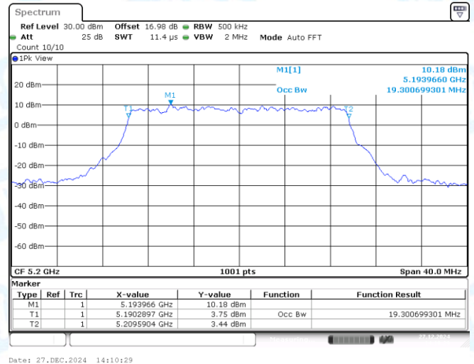
11AX20MIMO-Ant2-5200
