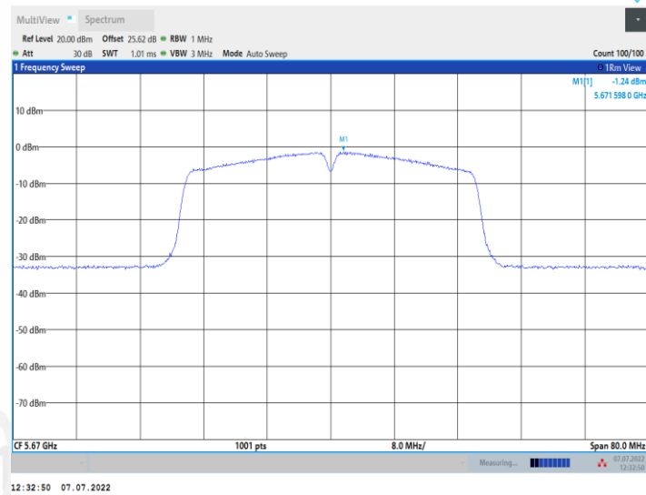
11N40MIMO_Ant2_5670
