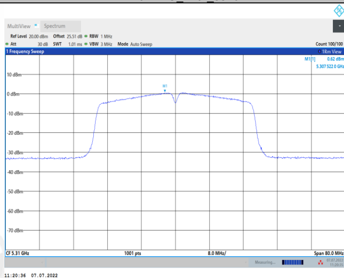
11N40MIMO_Ant2_5310
