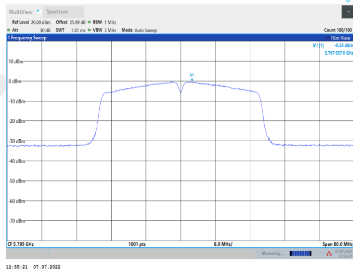
11N40MIMO_Ant2_5795
