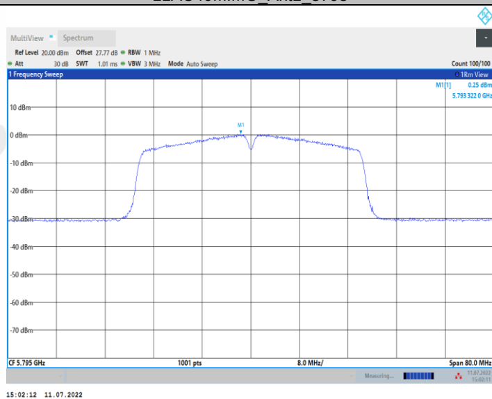
11AC40MIMO_Ant2_5795
