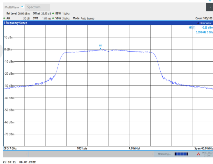
11N20MIMO_Ant2_5700
