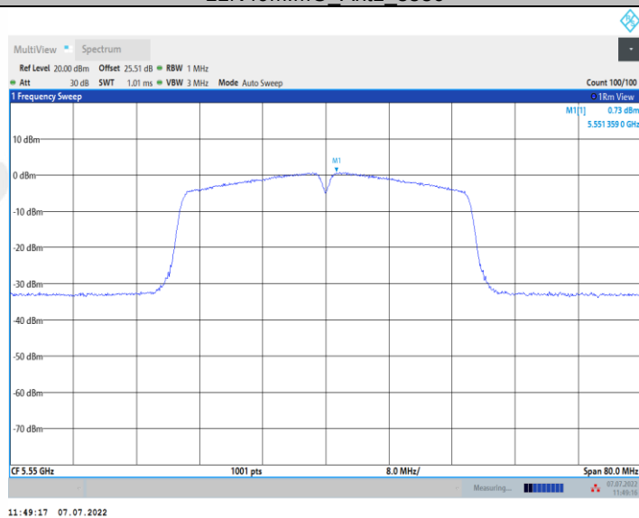
11N40MIMO_Ant2_5550
