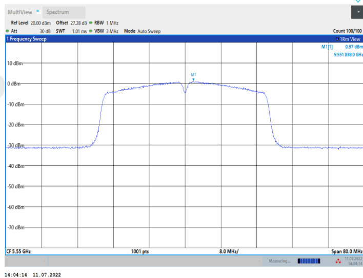
11AC40MIMO_Ant2_5550
