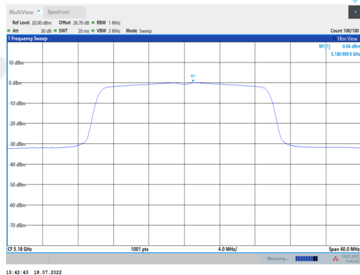
11AX20MIMO_Ant1_5180
