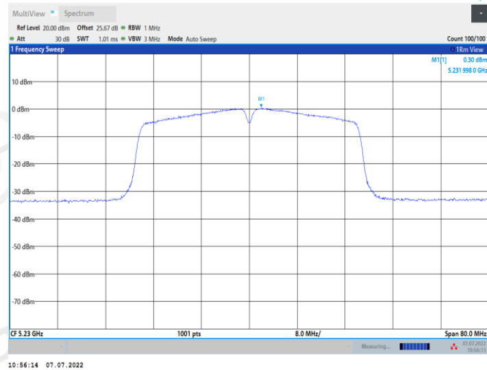
11N40MIMO_Ant2_5230
