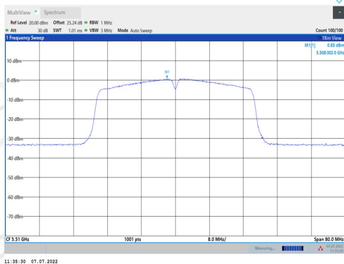
11N40MIMO_Ant2_5510
