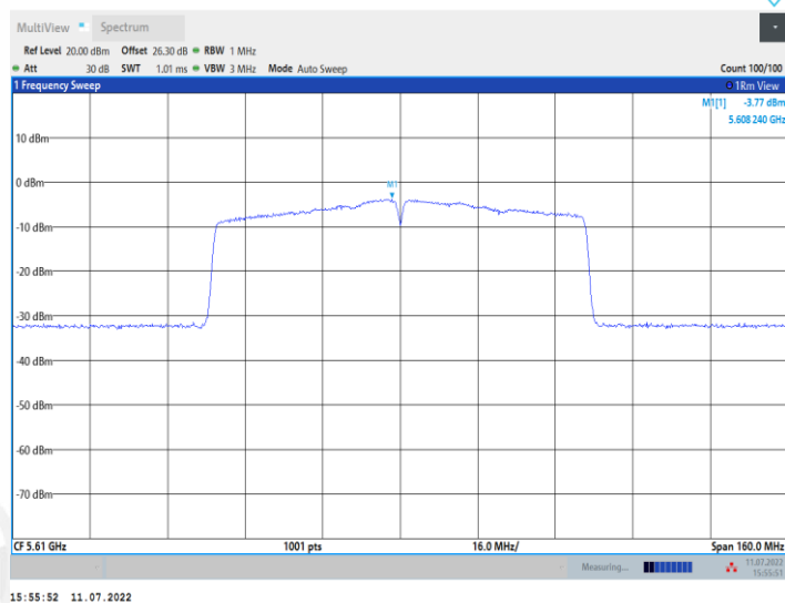
11AC80MIMO_Ant2_5610
