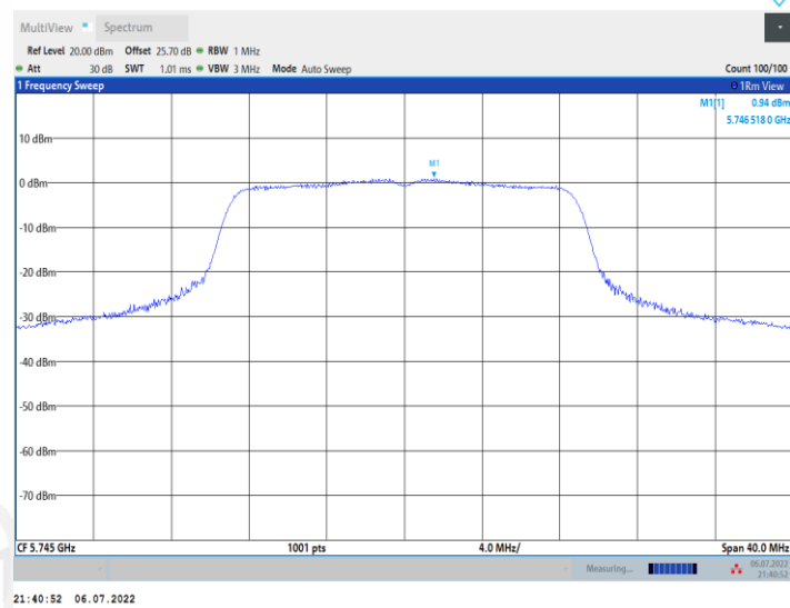
11N20MIMO_Ant2_5745
