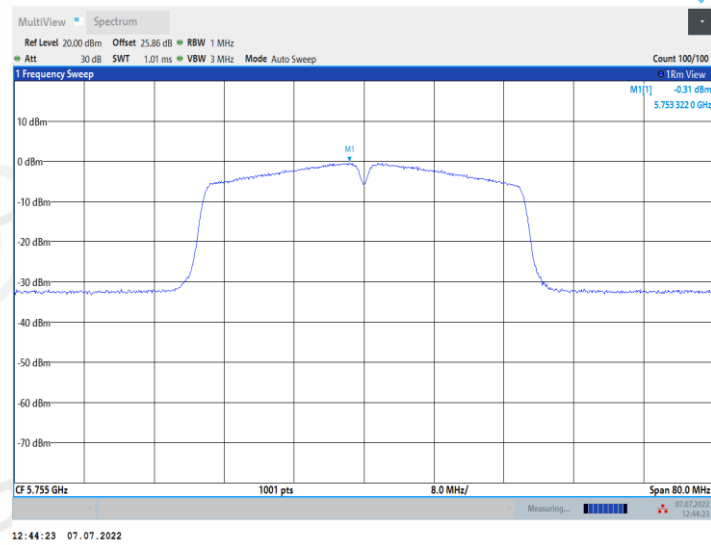
11N40MIMO_Ant2_5755
