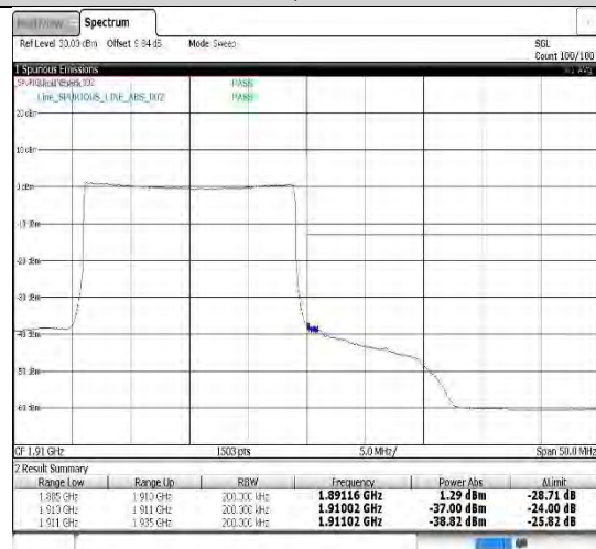
Band2-20MHz-16QAM-19100-100RB#0
