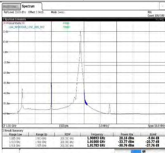
Band2-20MHz-16QAM-19100-1RB#99
