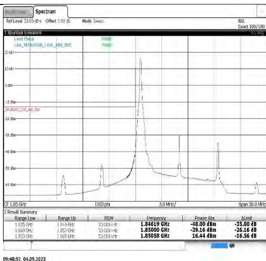
Band2-10MHz-QPSK-18650-50RB#0
