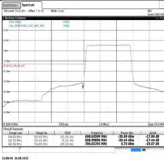
Band12-3MHz-QPSK-23165-15RB#0
