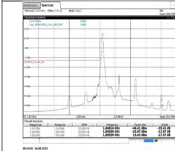
Band2-5MHz-16QAM-18625-1RB#0
