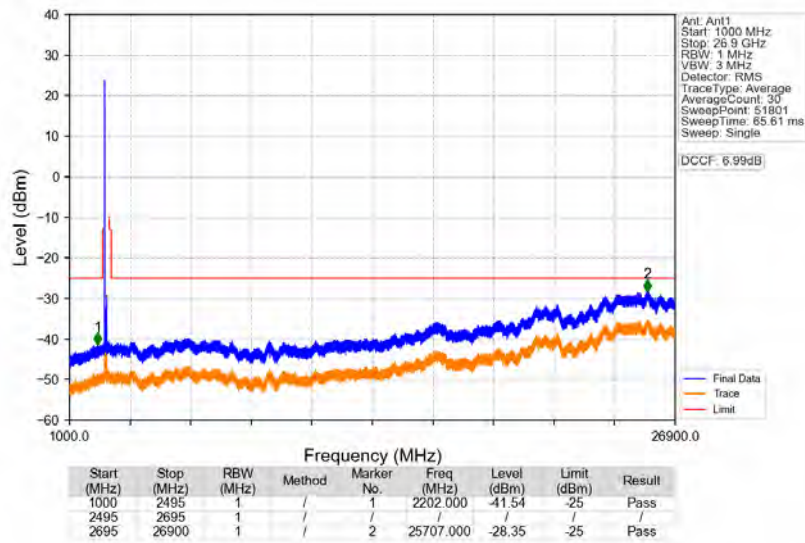
n41_30kHz_SISO_NTNV_90MHz_CP-OFDM_QPSK_2541MHz_Edge_1RB_Left
