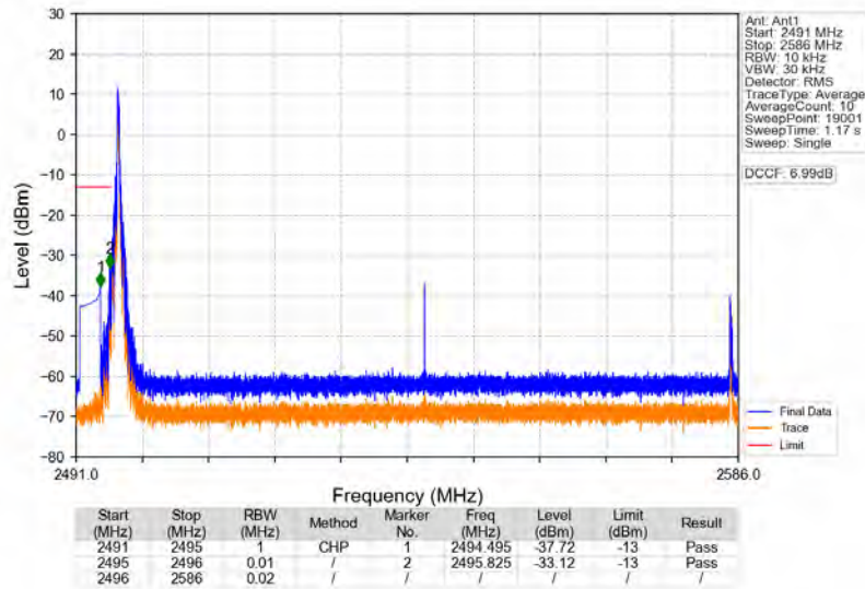
n41_30kHz_SISO_NTNV_90MHz_CP-OFDM_QPSK_2541MHz_Edge_1RB_Left
