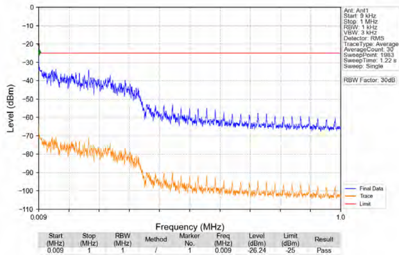
n41 30kHz SISO NTNV 90MHz CP-OFDM QPSK 2644.98MHz Edge 1RB Right
