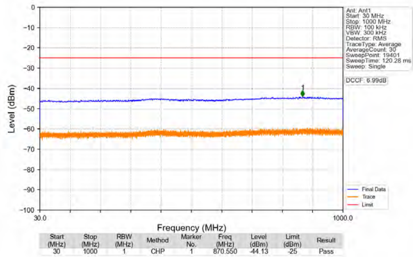
n41_30kHz_SISO_NTNV_90MHz_CP-OFDM_QPSK_2541MHz_Edge_1RB_Left
