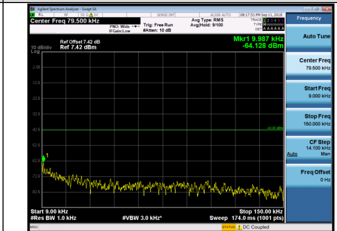
20MHz_LCH_QPSK_1RB#0
