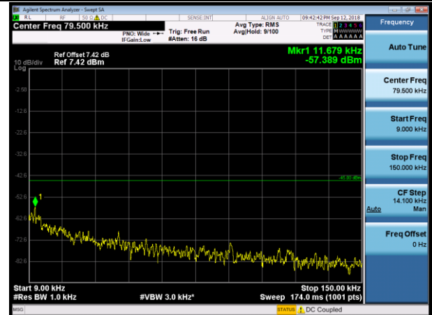
20MHz_LCH_QPSK_1RB#0
