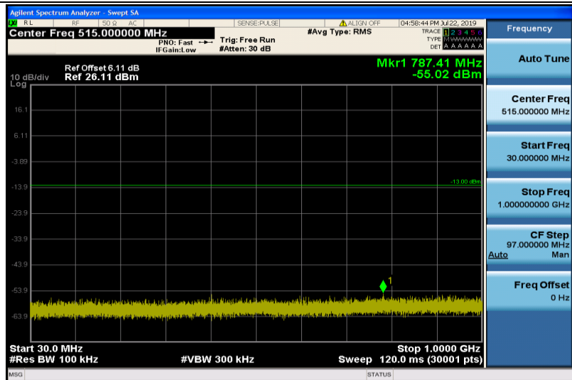
Band2-3MHz-QPSK-18615-1RB#0-30~1000MHz
