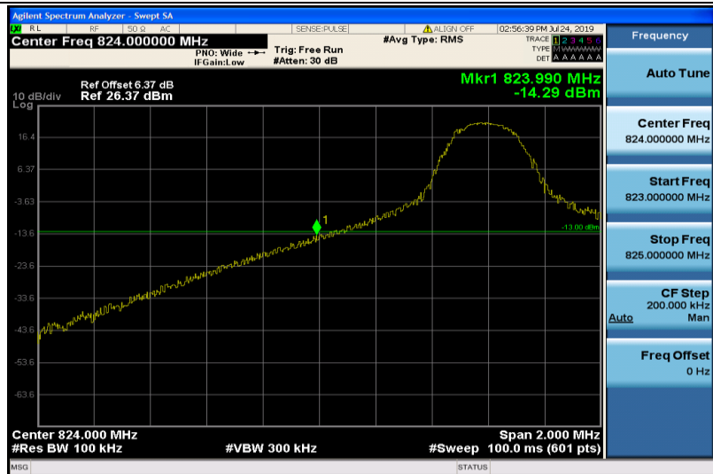
Band5-10MHz-QPSK-20450-1RB#0
