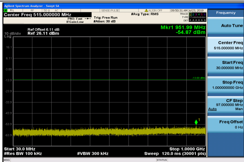
Band2-5MHz-QPSK-19175-1RB#0-30~1000MHz
