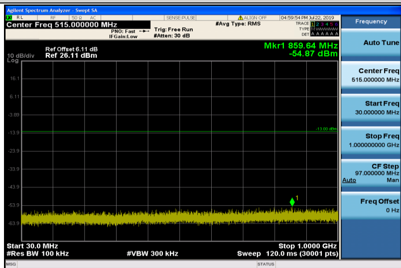
Band2-3MHz-QPSK-18900-1RB#0-30~1000MHz
