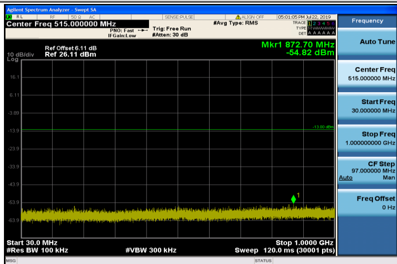
Band2-3MHz-QPSK-19185-1RB#0-30~1000MHz
