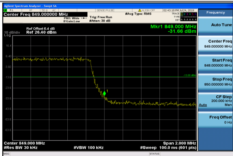
Band5-3MHz-QPSK-20635-15RB#0
