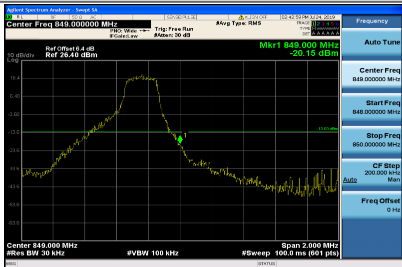
Band5-3MHz-QPSK-20635-1RB#14
