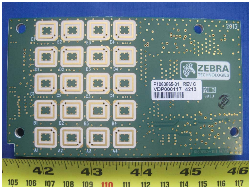
RFID module Bottom View
