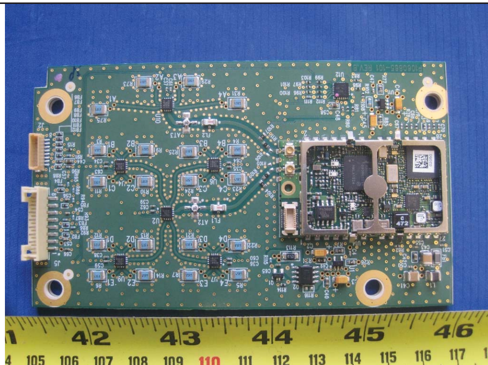
RFID module Top View
