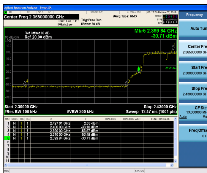
11N40SISO_Ant2_Low_2422
