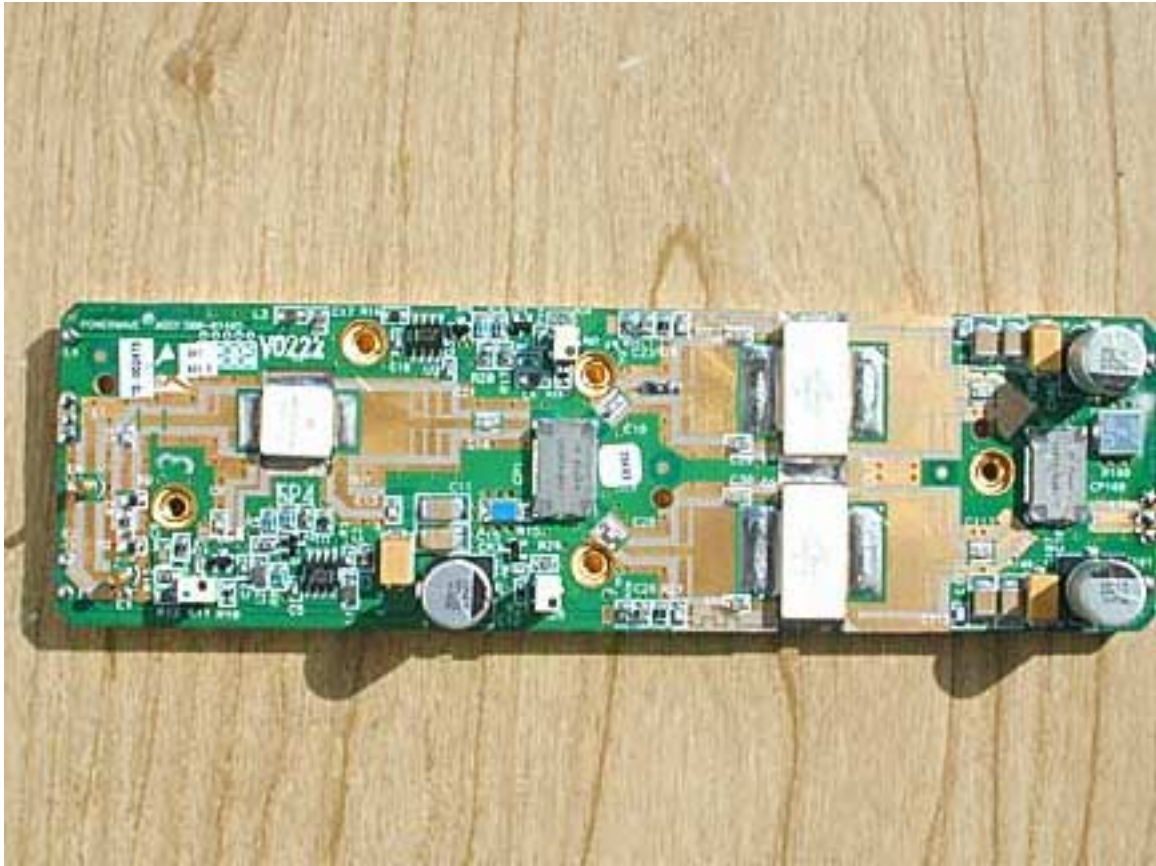
500-01405 PCB Top
