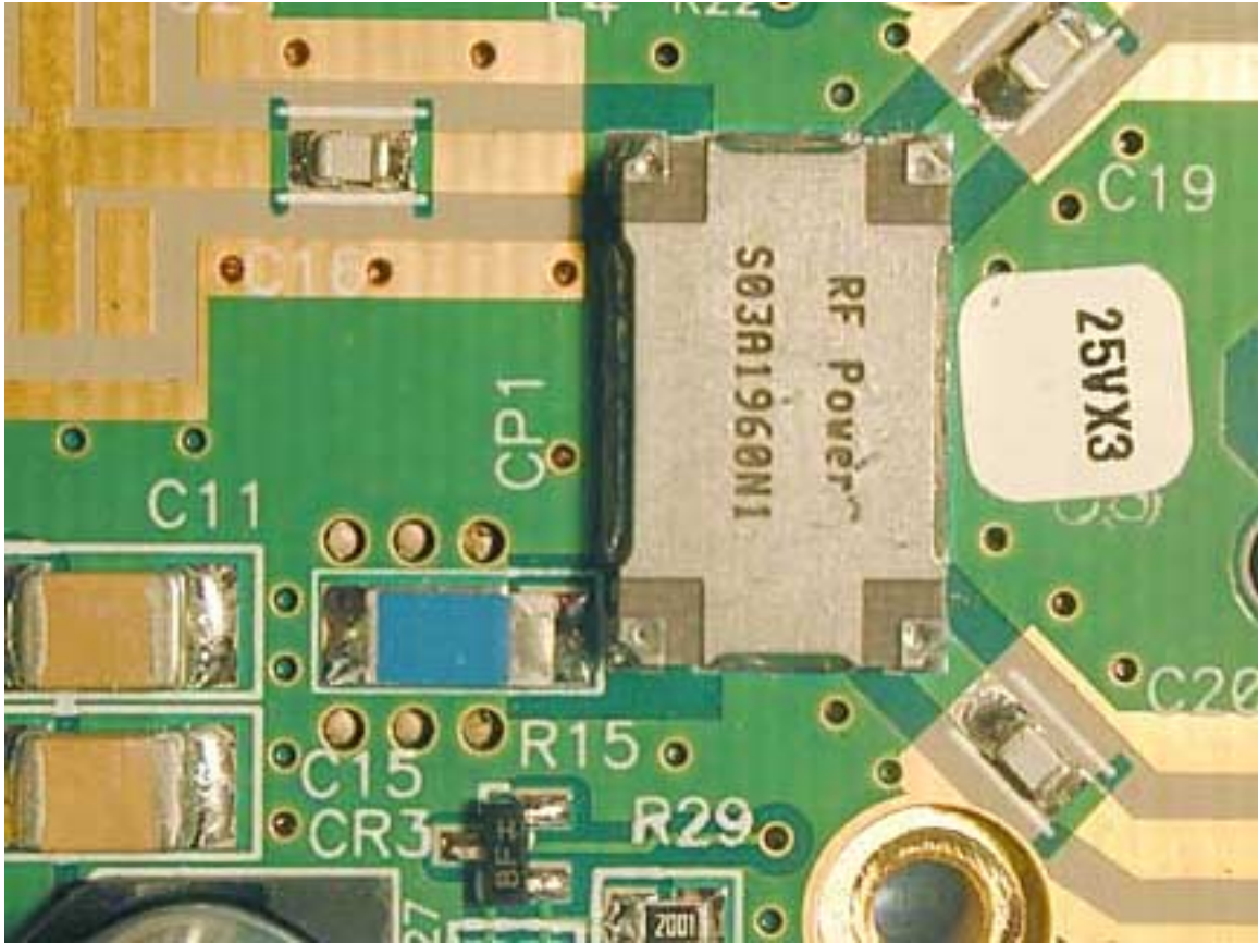
500-01405 RF Module 4
