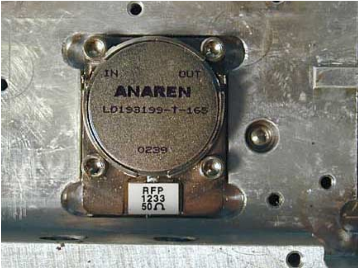
500-02215 RF Module
