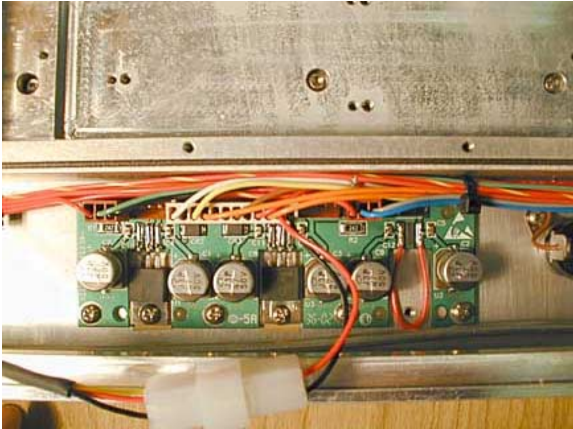
500-02230 PCB Top
