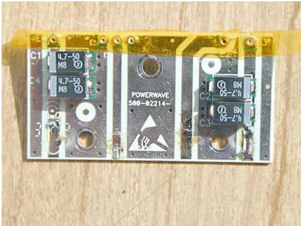
500-02214 PCB top
