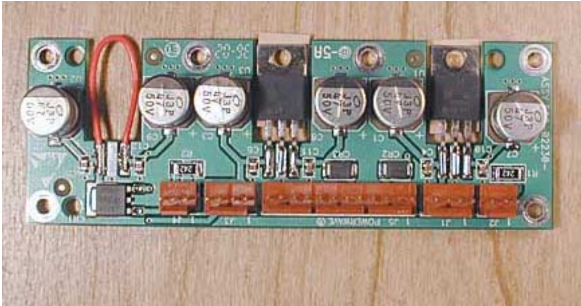
500-02230 PCB Top 2
