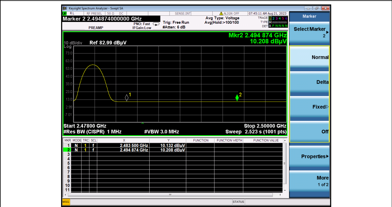
(AVERAGE, Channel 78, \pi/4 -DQPSK)
