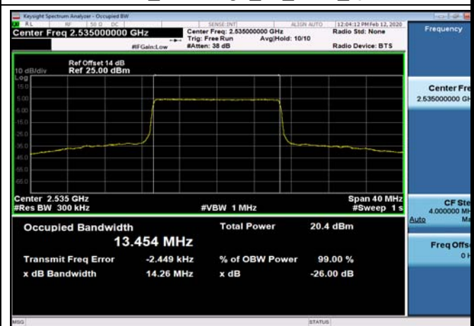
FDD07_MidRange_20_2535_Q16
