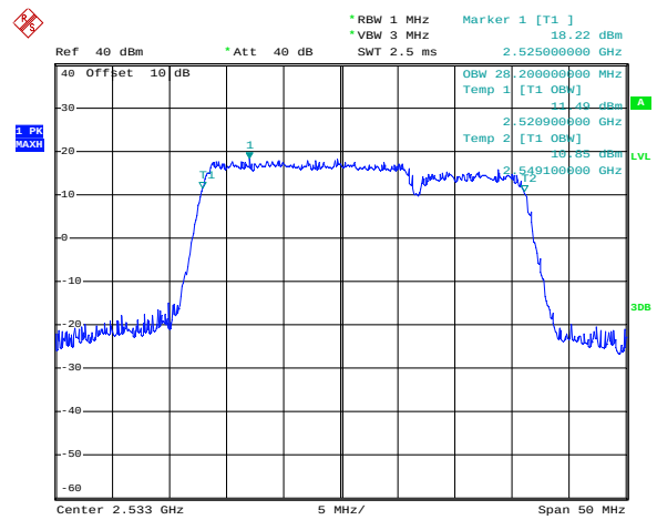
FDD7_MidRange_20+10_Q16
