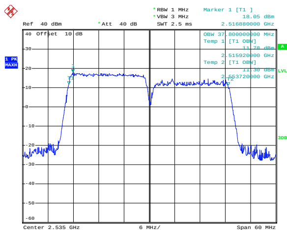
FDD7_MidRange_20+20_QPSK
