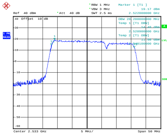
FDD7_MidRange_20+10_QPSK
