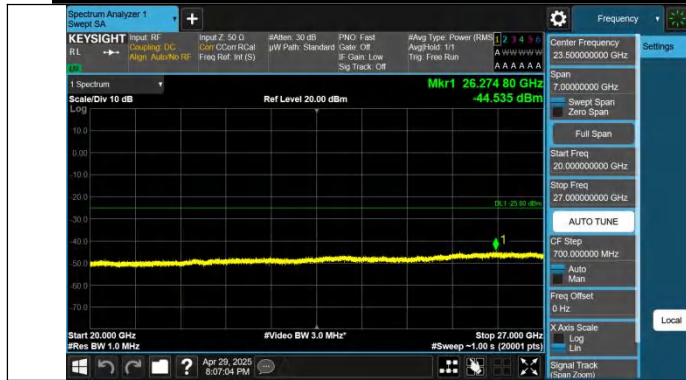
Band7-15MHz-QPSK-20825-1RB#0-20000~27000-PASS
