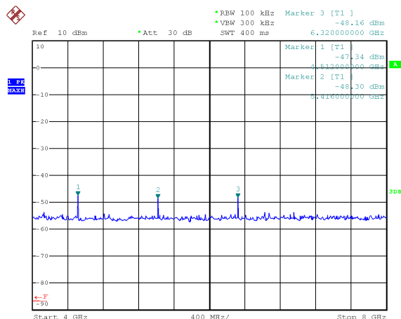
Plot 5 (4÷8GHz)
