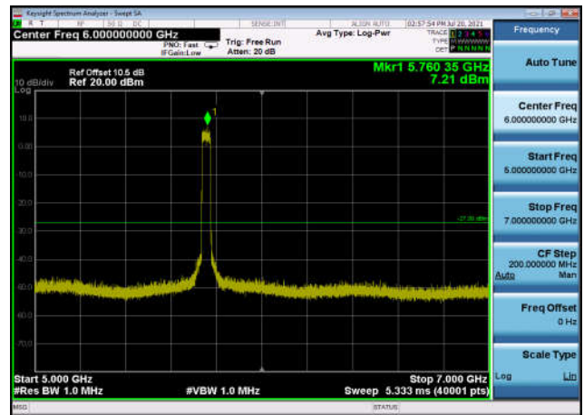
U-NII-3 ,Plot 3,5000MHz~7000MHz-802.1 1ax(80MHz),5775MHz,Ant1
