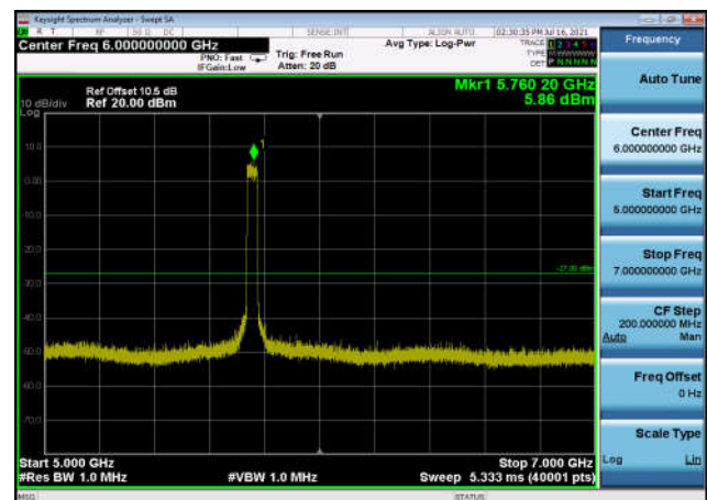
U-NII-3 ,Plot 3,5000MHz~7000MHz-802.1 1ax(40MHz),5755MHz,Ant0
