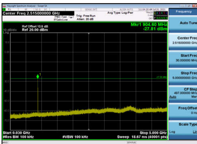
U-NII-3 ,Plot 2,30MHz~5000MHz-802.11a x(20MHz),5745MHz,Ant1
