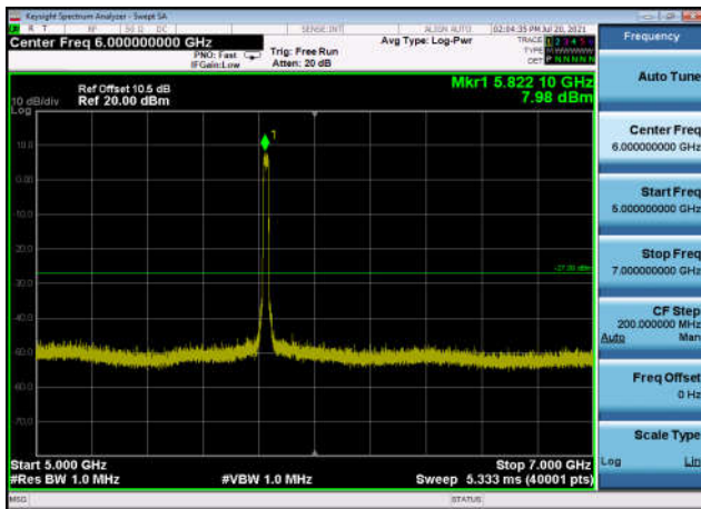
U-NII-3 ,Plot 3,5000MHz~7000MHz-802.1 1ax(40MHz),5795MHz,Ant1
