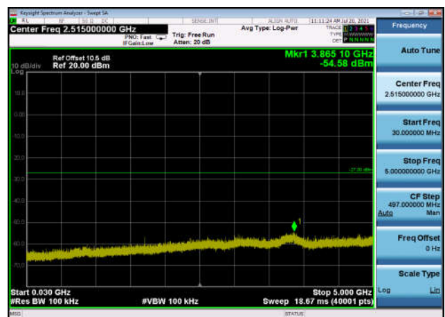
U-NII-3 ,Plot 2,30MHz~5000MHz-802.11a x(20MHz),5785MHz,Ant1
