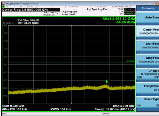
U-NII-3 ,Plot 2,30MHz~5000MHz-802.11a x(40MHz),5795MHz,Ant1
