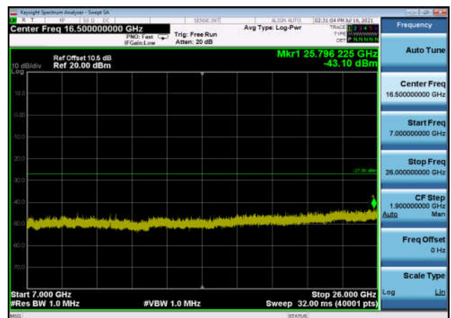
U-NII-3 ,Plot 4,7000MHz~26000MHz-802. 11ax(40MHz),5755MHz,Ant0
