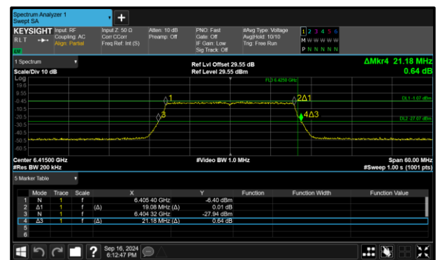
Figure 34 - 802.11ax HE20 SU LPI Maximum 99% OBW
