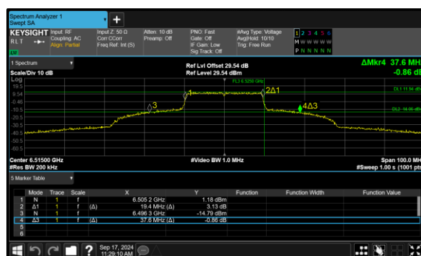
Figure 44 - 802.11ax HE20 SU SP Maximum 99% OBW
