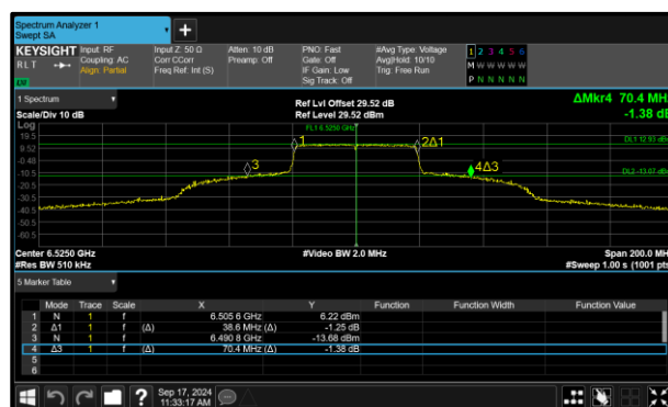
Figure 46 - 802.11ax HE40 SU SP Maximum 99% OBW
