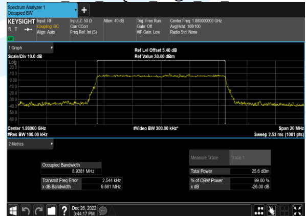
B2 10M 64QAM 50@0 CH 18900
