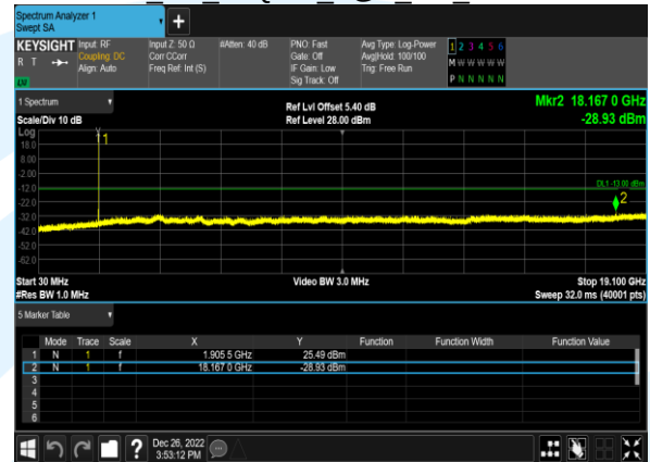
B2 3M 64QAM 1@0 CH 18900
